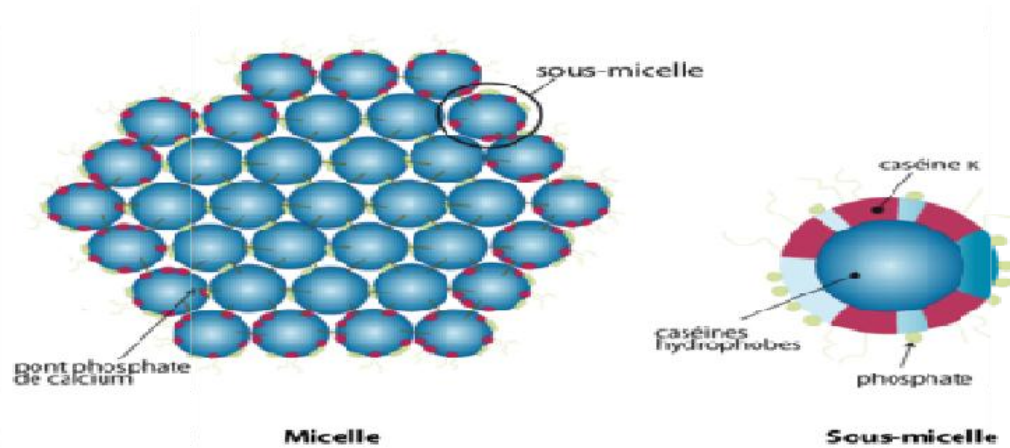
Figure N°2 : Représentation de la micelle de caséine avec sous-unités selon le modèle de Schmidt (1989)
