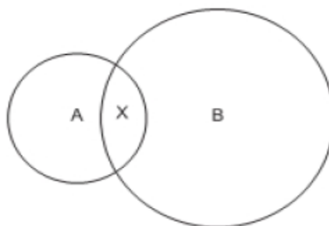
Figure II.6 : Atomes A, B et la zone de recouvrement X.
