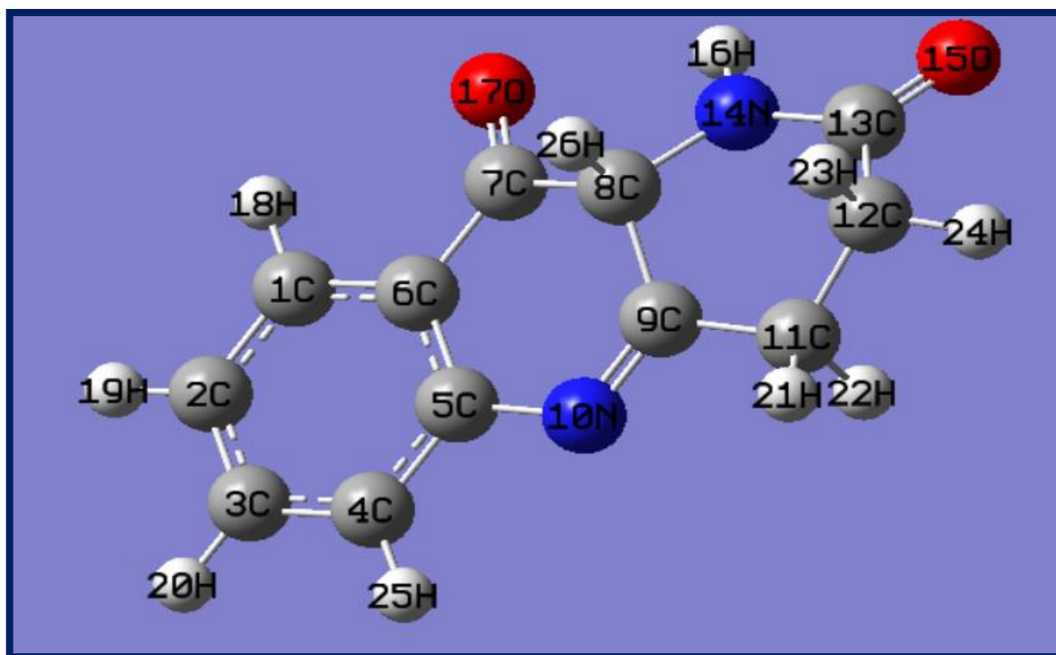
Figure IV.1 : Structure de la molécule quinazolinone optimisée par DFT B3LYP/6-31Gd
