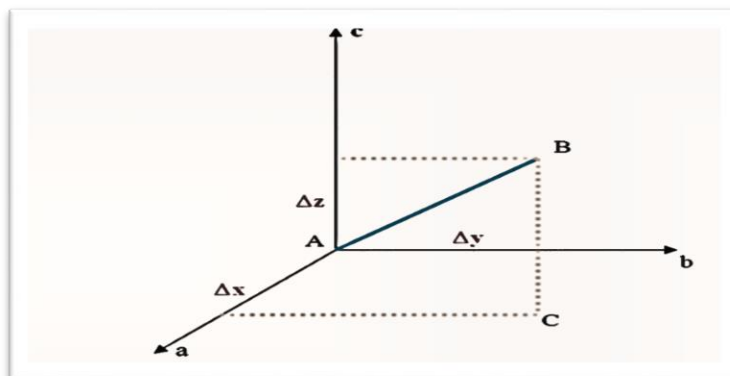
Figure IV.3 : Représentation des distances interatomiques.
