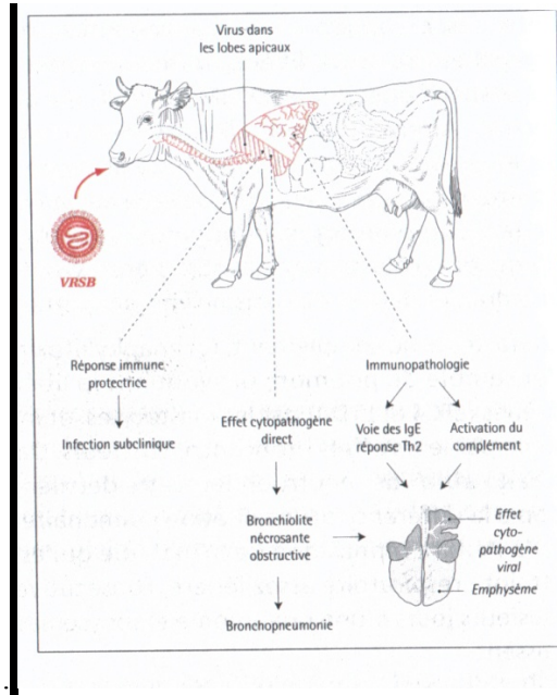
Schéma 19 : la pathogénie de VRSB (42)
