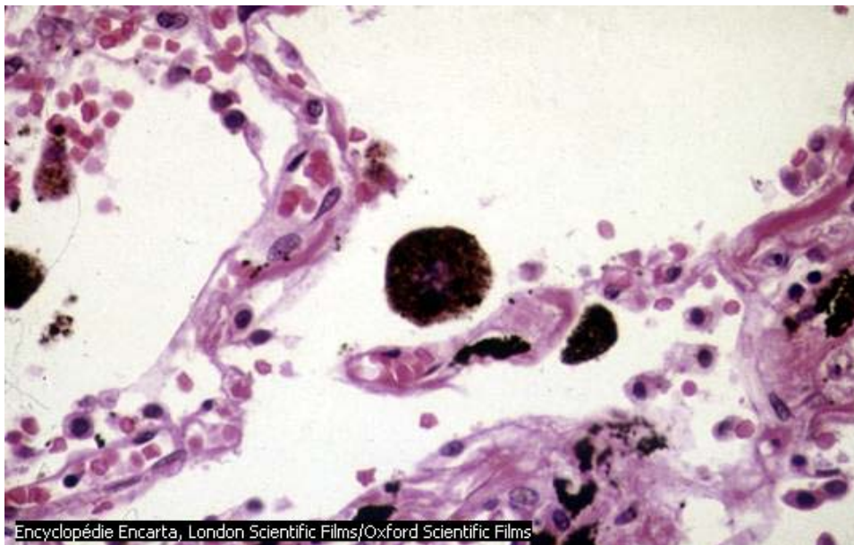
Schéma 12 : Aspect microscopique de l'emphysème
