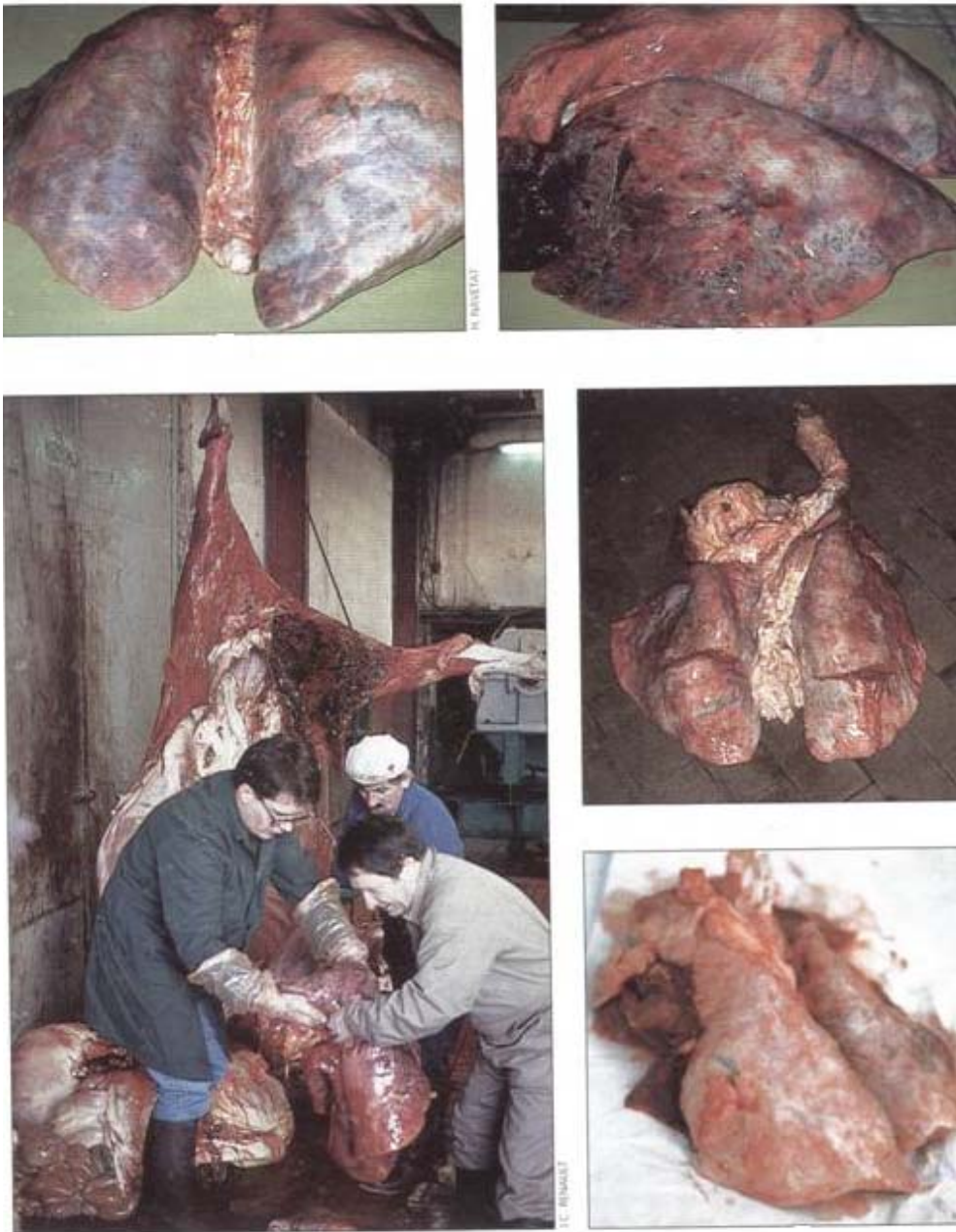
Schéma 13 : Les lésions d'emphyème pulmonaire
