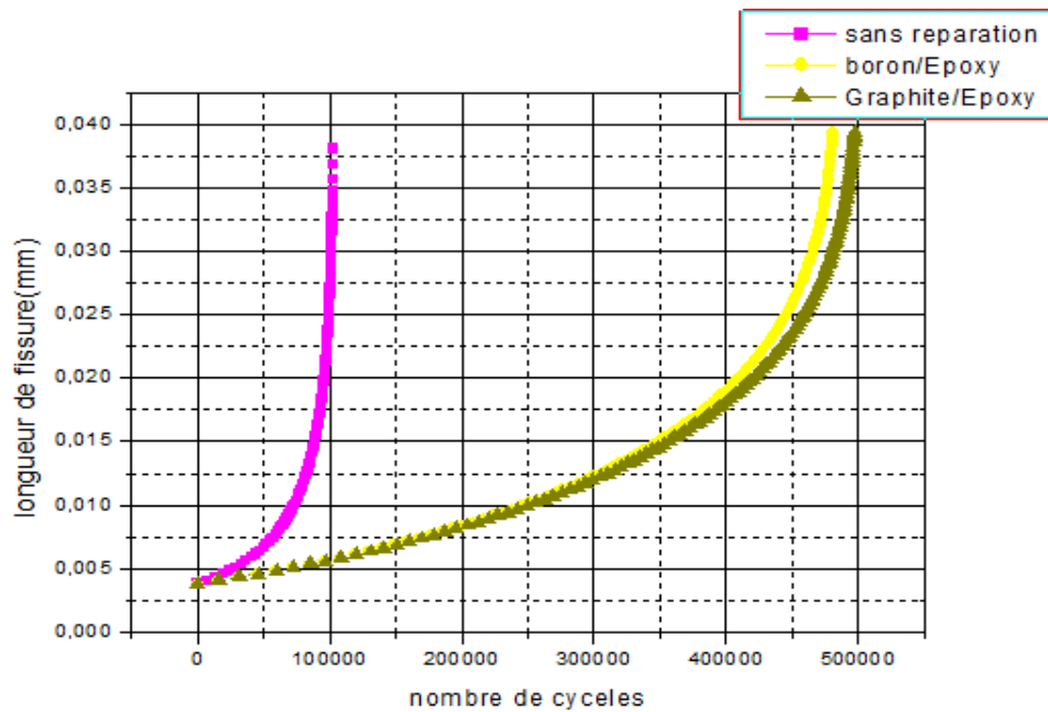
Figure III.28: Effet du matériau AL 2024-T3 sur la variation de la durée de vie sur la propagation de fissure pour la plaque non réparée et réparée par le Bore/Epoxy et graphite/Epoxy.
