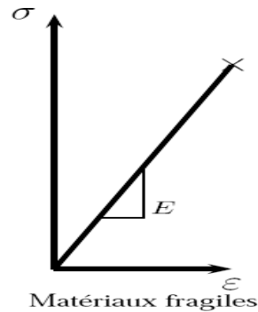
Figure I.8: Matériaux fragiles
