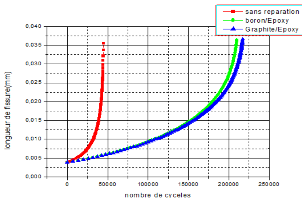
Figure III.13: Variation de la propagation de fissure en fonction du nombre de cycles de la plaque non réparée et réparée par le Bore/Epoxy et le graphite/Epoxy pour P=100 MPa.
