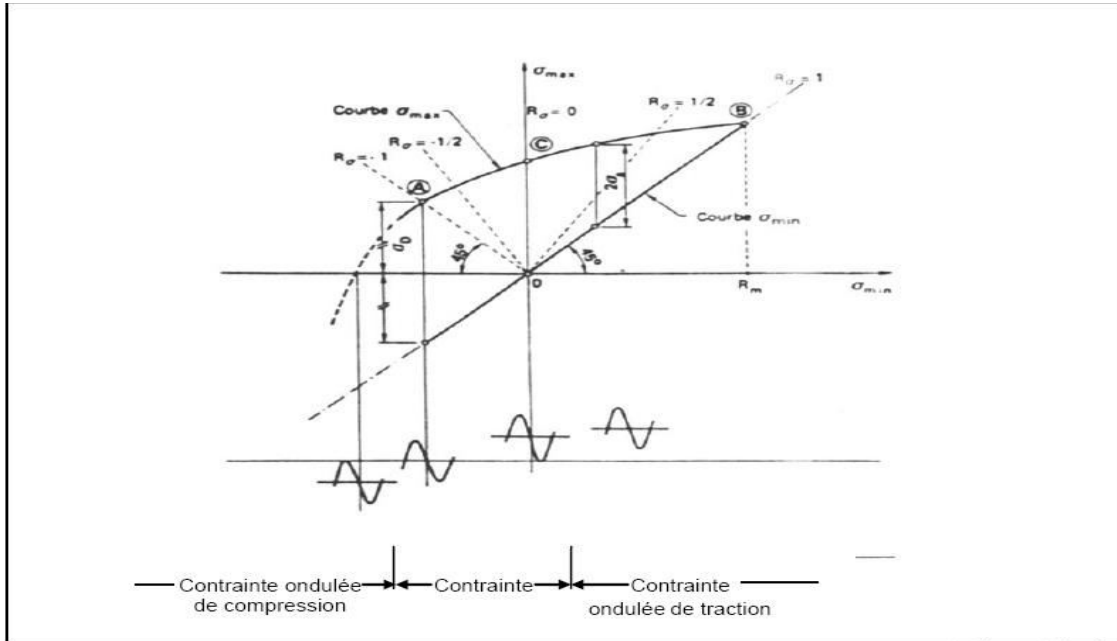
Figure I.15 : Diagramme de Ros
