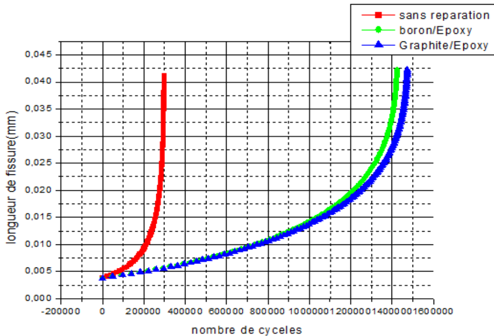
Figure III.15 : Variation de la propagation de fissure en fonction du nombre de cycles de la plaque non réparée et réparée par le Bore/Epoxy et le graphite/Epoxy pour P=60 MPa.
