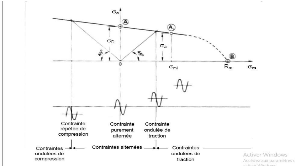
Figure I.13. : Diagramme de Haigh (résultats théorique)
