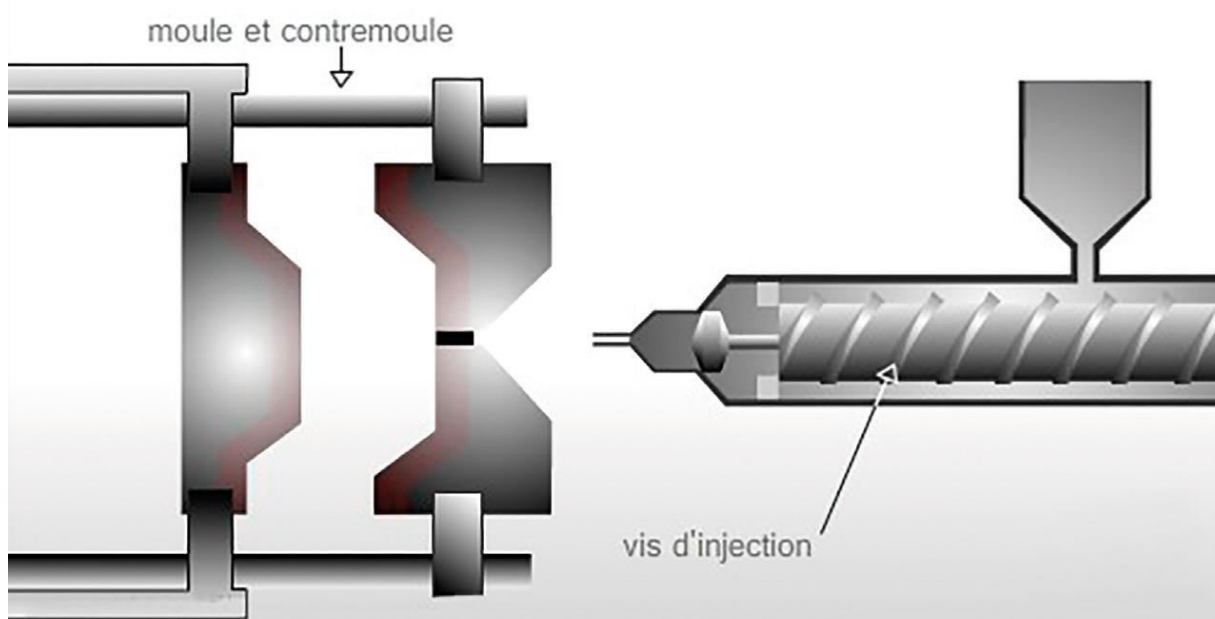
Figure II.11: Injection thermodurcissable BMC
