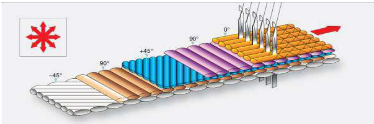
Figure II.5: Représentation schématique d'un stratifié multidirectionnel
