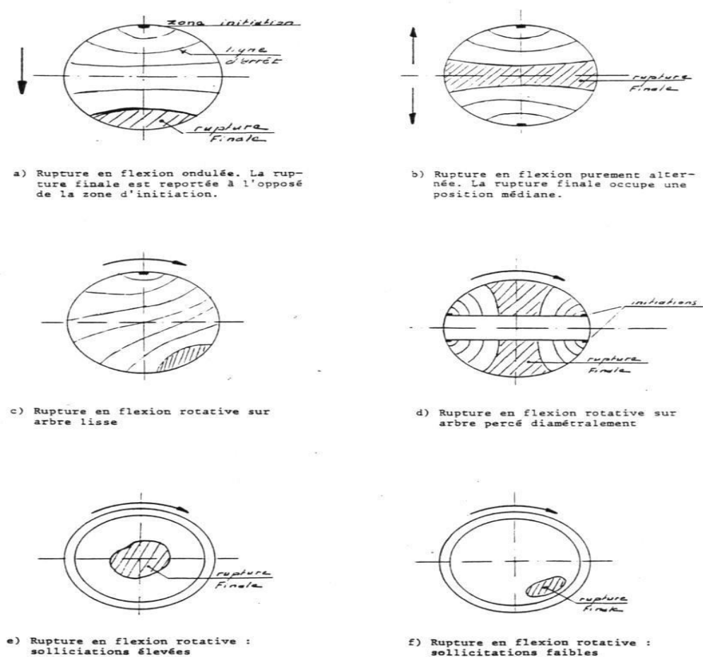
Figure I.19 : Faciès de fatigue
