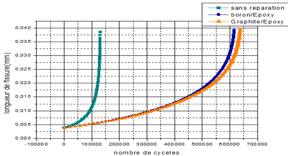
Figure III.17. : Variation de la propagation de fissure en fonction du nombre de cycles de la plaque non réparée et réparée par le Bore/Epoxy et le graphite/Epoxy pour R=0.2 .
