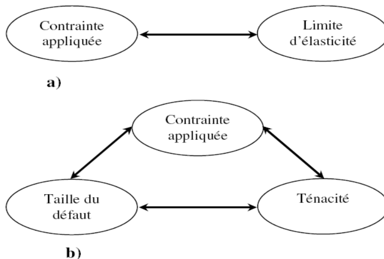
Figure I.5 : Comparaison de l'approche classique (a) et de l'approche utilisant la MRL
