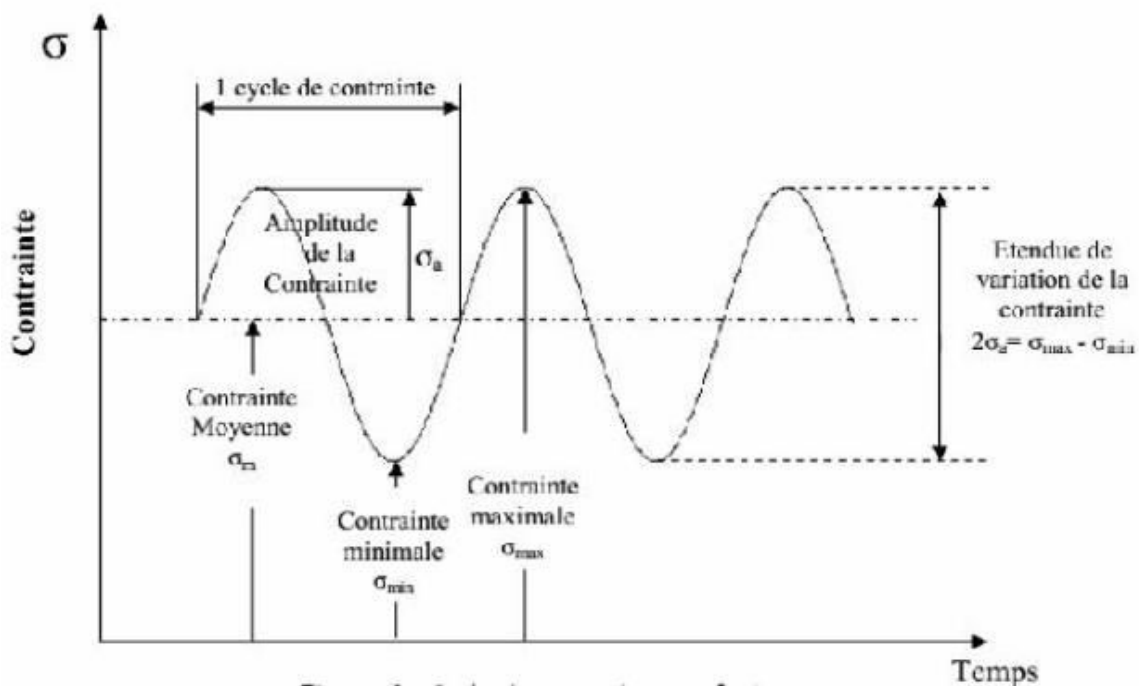
Figure I.17 : Cycle de contrainte en fatigue.
