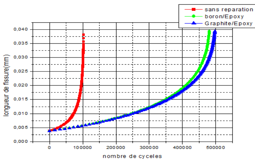
Figure III.14 : Variation de la propagation de fissure en fonction du nombre de cycles de la plaque non réparée et réparée par le Bore/Epoxy et le graphite/Epoxy pour P=80 MPa
