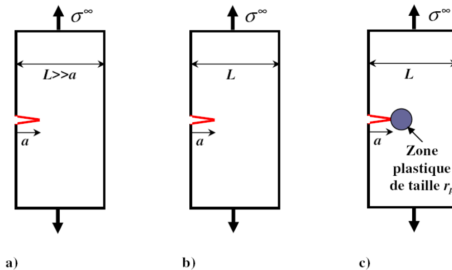
Figure I.23: Différents cas d'éprouvettes avec fissure de bord.
