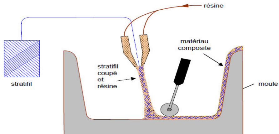
Figure II.10 : Moulage par projection simultanés
