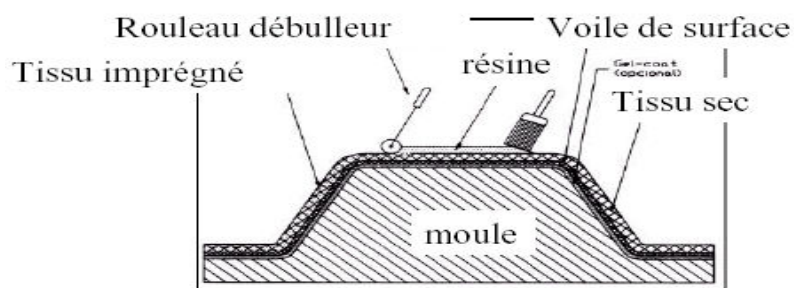
Figure II.9 : Moulage par contacts
