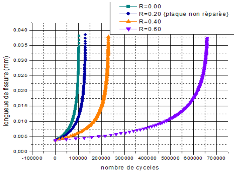
Figure III.20: Effet du rapport de charge sur la durée de vie en fatigue pour la plaque non réparée.
