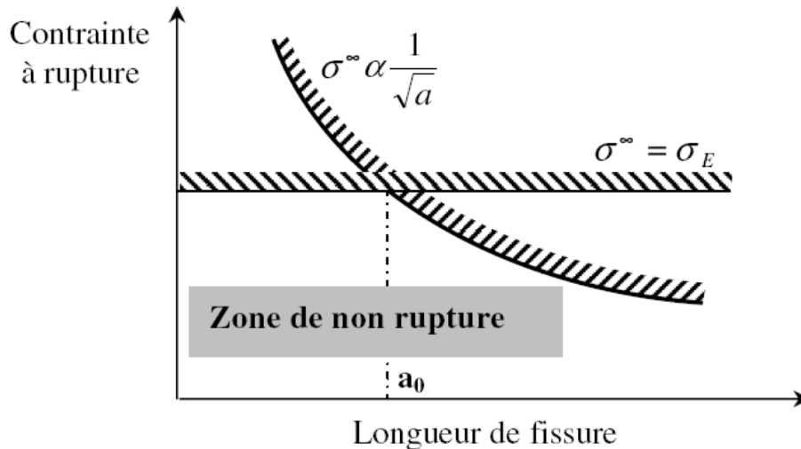
Figure I.22 : Comparaison entre l'approche classique et celle de la MLR.
