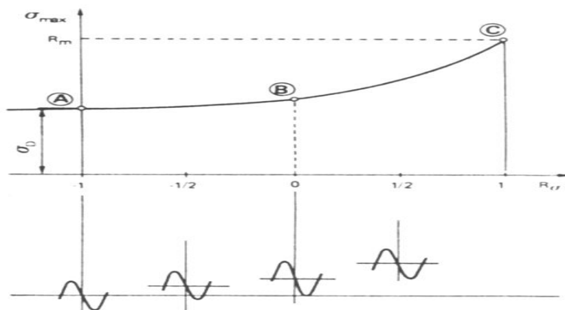
Figure I.16 : Diagramme de Moore-Kommers- Jaspers
