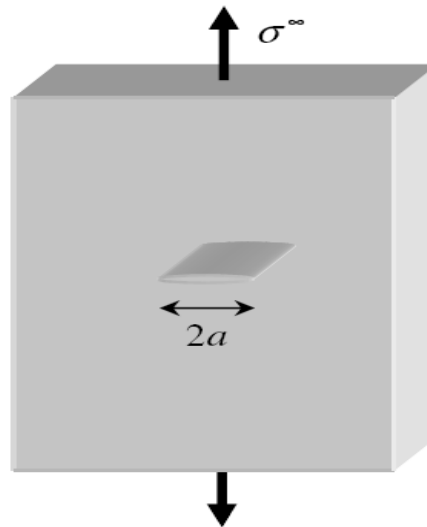
Figure I.21 : Fissure traversant de longueur 2a dans une plaque infinie
