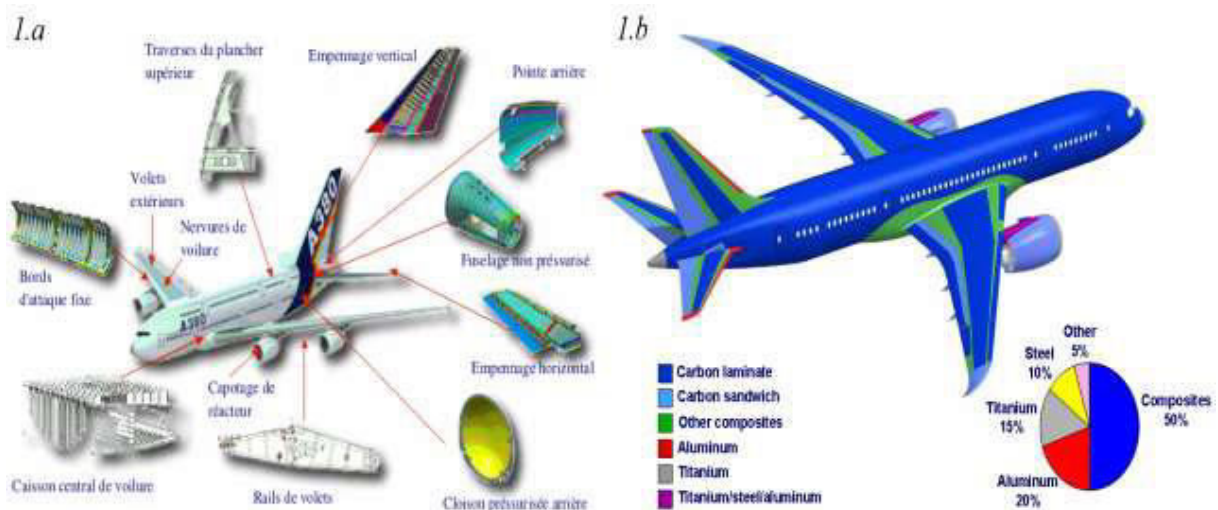
Figure II.14: Répartition des matériaux composites dans l'A380 (a) (source Airbus) et dans Boeing B787, (b) (source Boeing).
