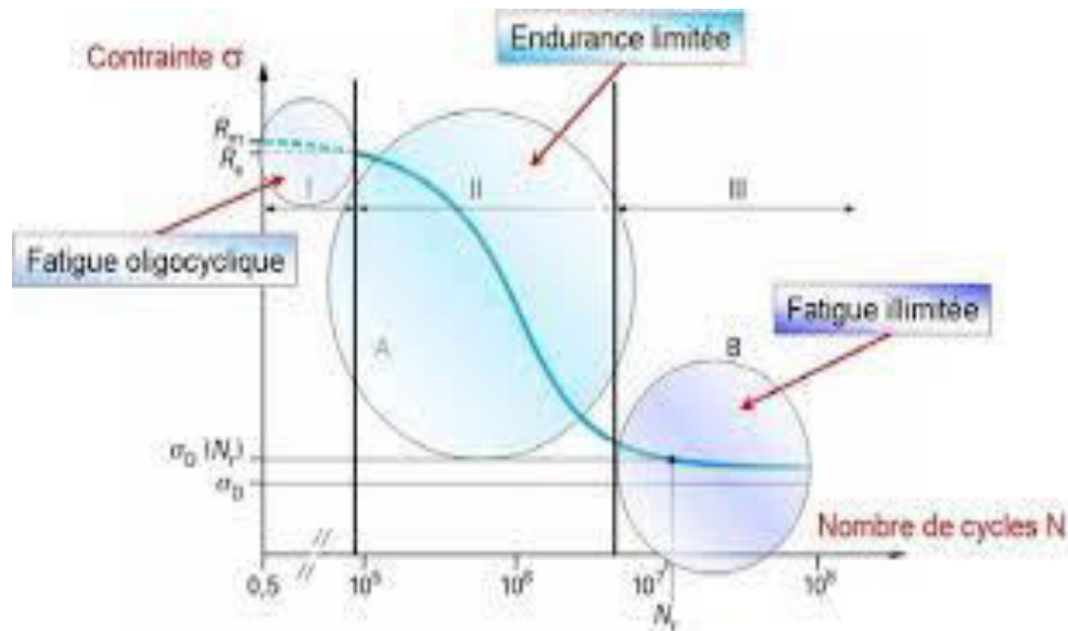
Figure I.11: Allure de la courbe de Wöhler
