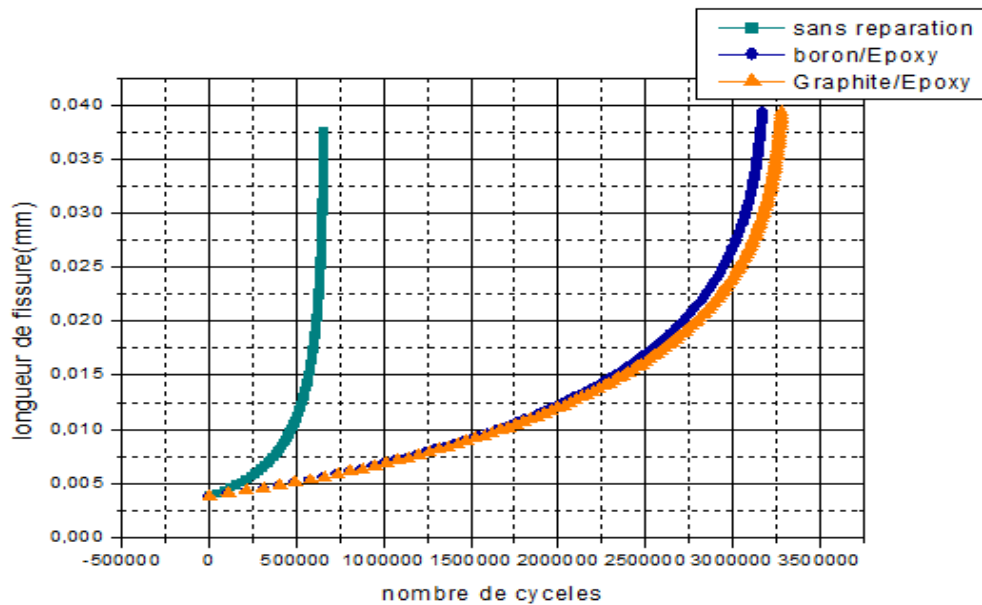
Figure III.19 : Variation de la propagation de fissure en fonction du nombre de cycles de la plaque non réparée et réparée par le Bore/Epoxy et le graphite/Epoxy pour R=0.6 .
