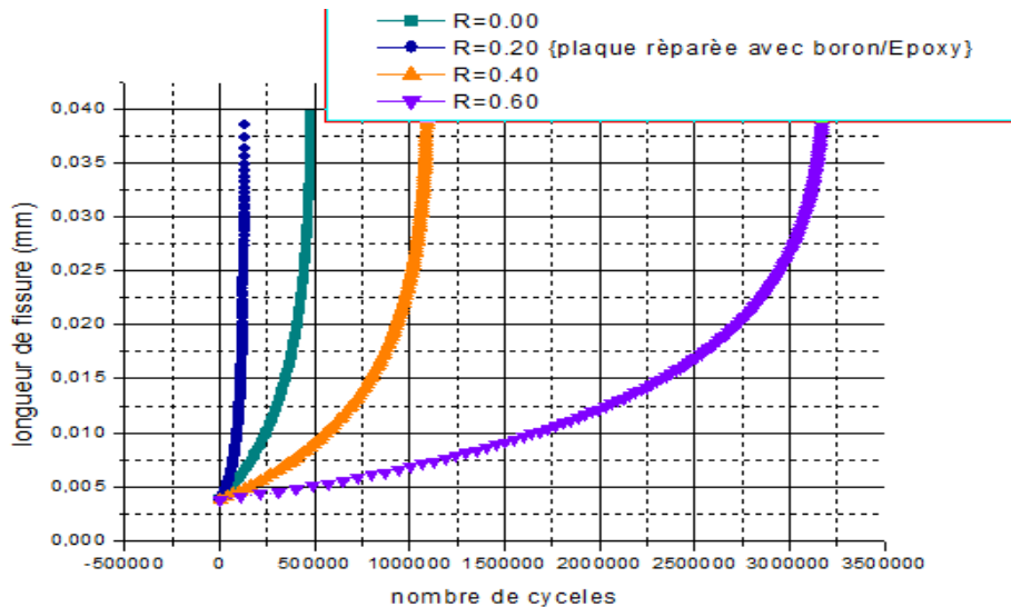
Figure III.22: Effet du rapport de charge sur la durée de vie en fatigue pour la plaque réparée par le patch Bore/Epoxy.
