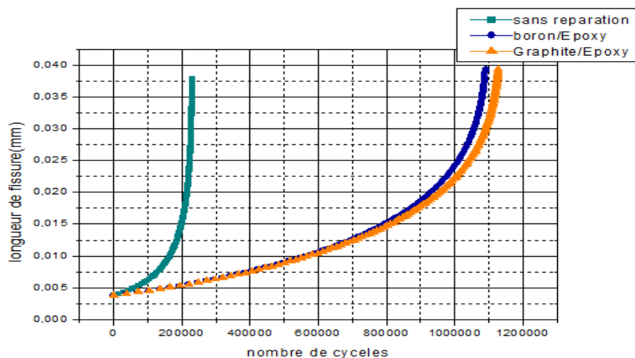
Figure III.18 : Variation de la propagation de fissure en fonction du nombre de cycles de la plaque non réparée et réparée par le Bore/Epoxy et le graphite/Epoxy pour R=0.4 .
