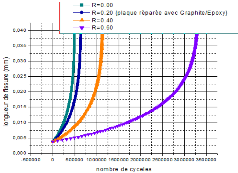
Figure III.21: Effet du rapport de charge sur la durée de vie en fatigue pour la plaque réparée par le patch graphite/époxy.
