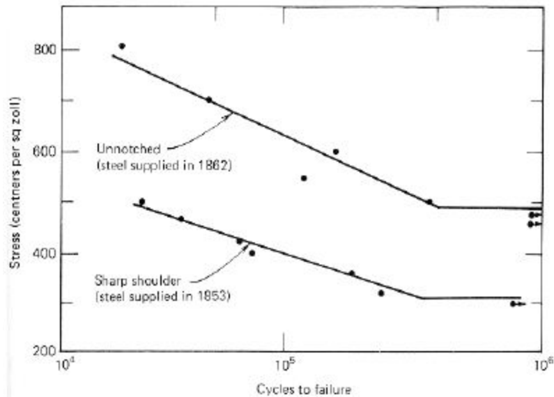
Figure I.2 (b) : courbe de Wöhler
