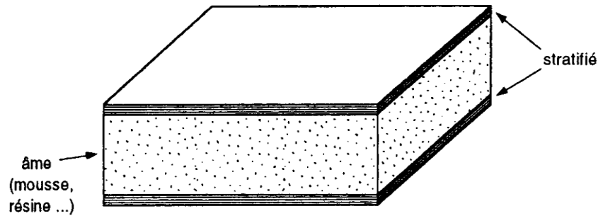
Figure II.8: Matériaux composite à âmes pleines.
