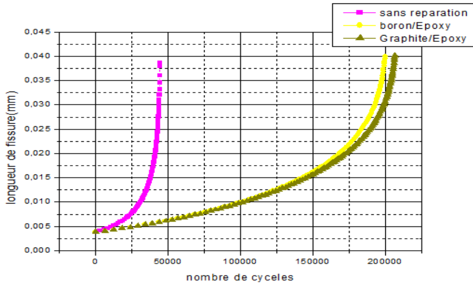
Figure III.26 : Effet du matériau AL 2024-T861 sur la variation de la durée de vie sur la propagation de fissure pour la plaque non réparée et réparée par le Bore/Epoxy et graphite/Epoxy.
