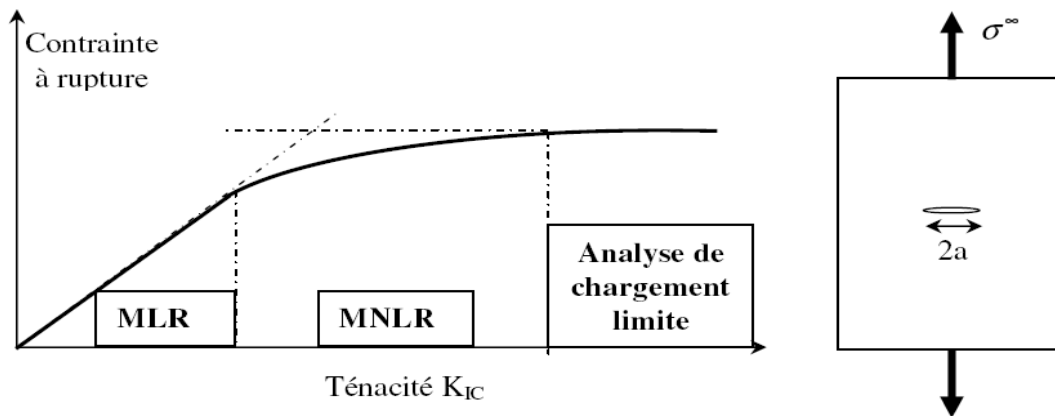
Figure I.20 : Comportement en fonction de la ténacité.
