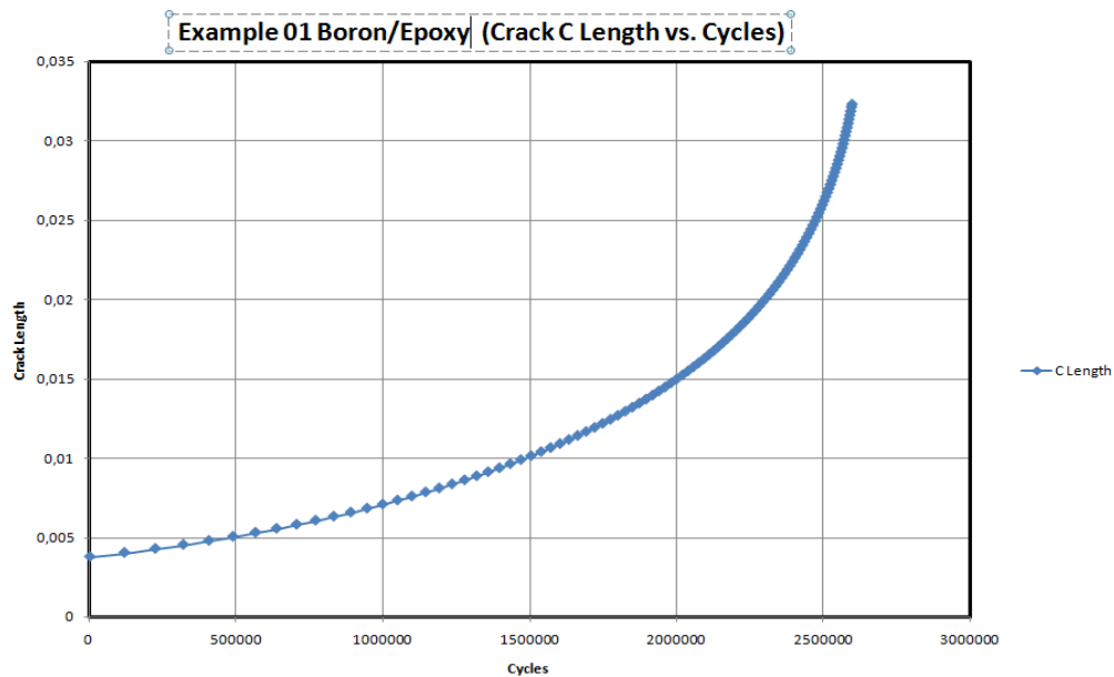
Figure III.10 : Variation de la propagation de fissure en fonction du nombre de cycles de la plaque réparée par le composite Bore/Epoxy.
