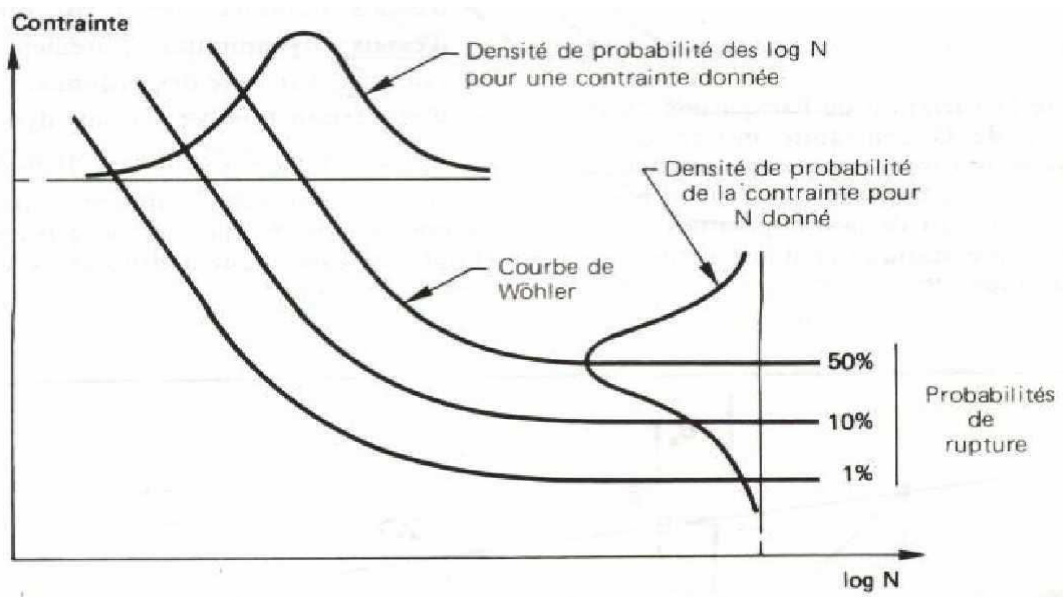
Figure I.12. : Courbe d'équiprobabilité de rupture (résultats théoriques)
