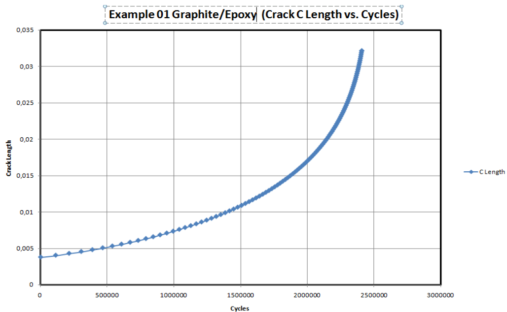
Figure III.12: Variation de la propagation de fissure en fonction du nombre de cycles de la plaque réparée par le composite Graphite/Epoxy.
