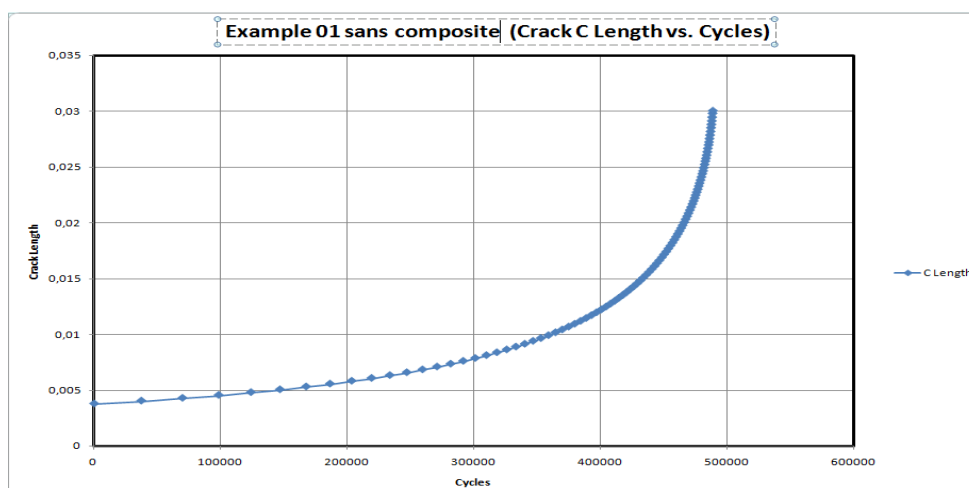
Figure III. 5: Variation de la longueur de fissure en fonction du nombre de cycles pour la plaque non réparée.
