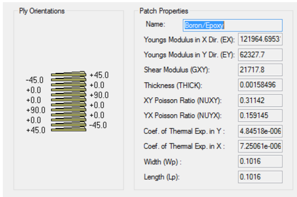
Figure III.7 : Interface des différentes propriétés et les différentes orientations du Bore/Epoxy.
