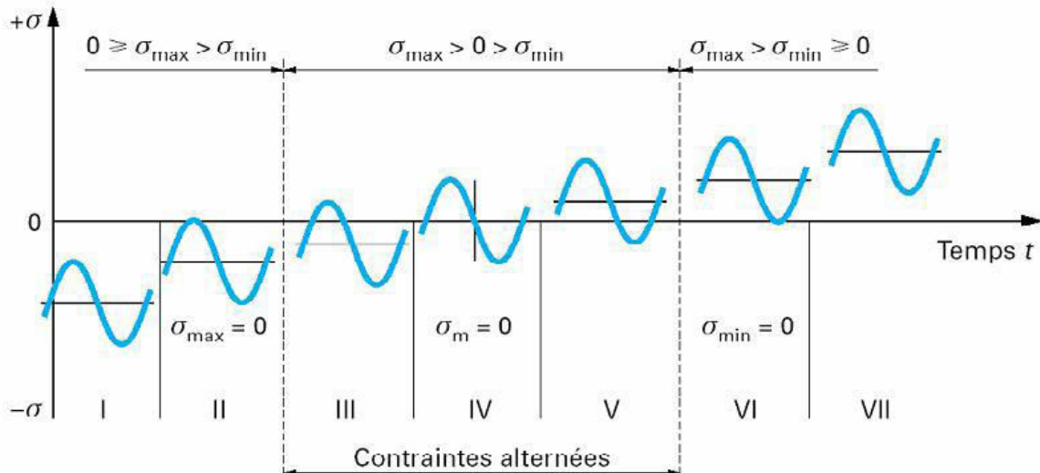
Figure I.18 : Les différentes formes de cycle de contrainte au cours d'essai de fatigue (Rabbe et al.2000)
