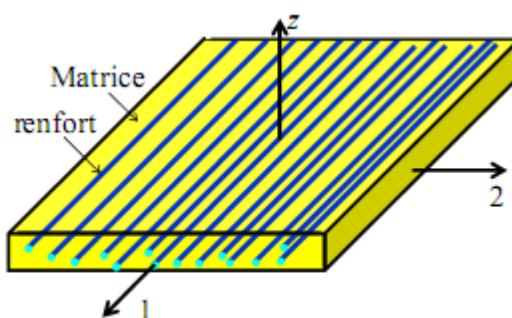
Figure II.4 : Représentation schématique d'un pli
