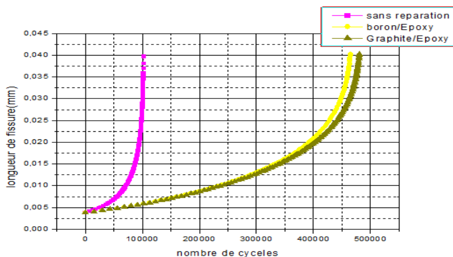
Figure III.24 : Effet du matériau AL 2024-T62 sur la variation de la durée de vie sur la propagation de fissure pour la plaque non réparée et réparée par le Bore/Epoxy et graphite/Epoxy.
