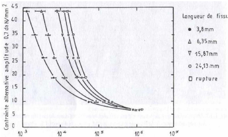
Figure I.7 : Courbe de fissuration donnant la longueur de la fissure selon la nombre de cycles et le niveau de contrainte
