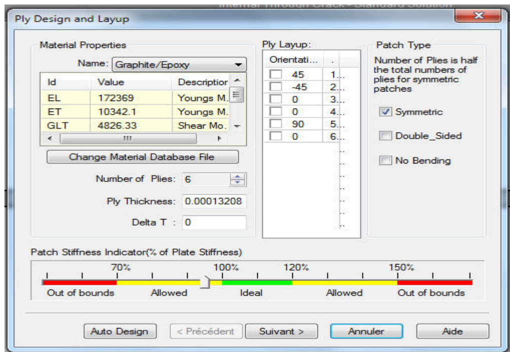
Figure III.11: Interface des propriétés et le nombre de plies et leurs orientations du patch Graphite/Epoxy.
