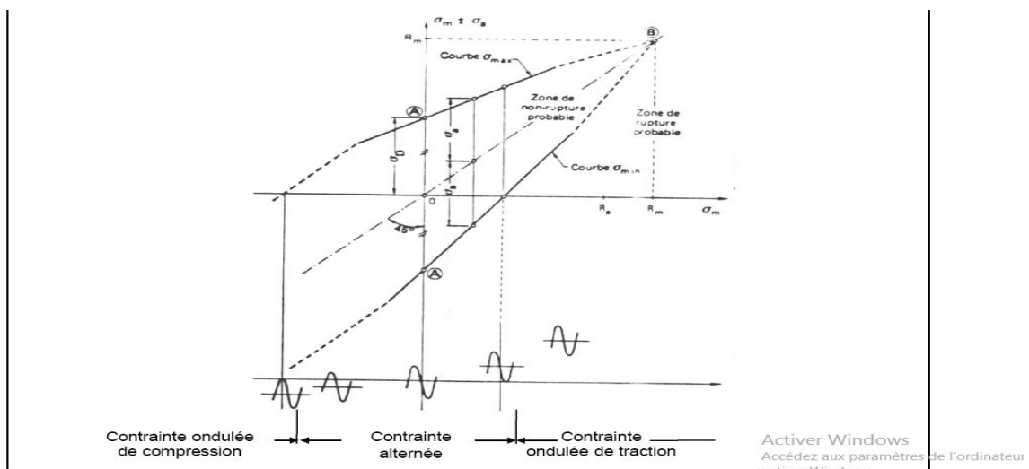
Figure I.14. : Diagramme de Goodman
