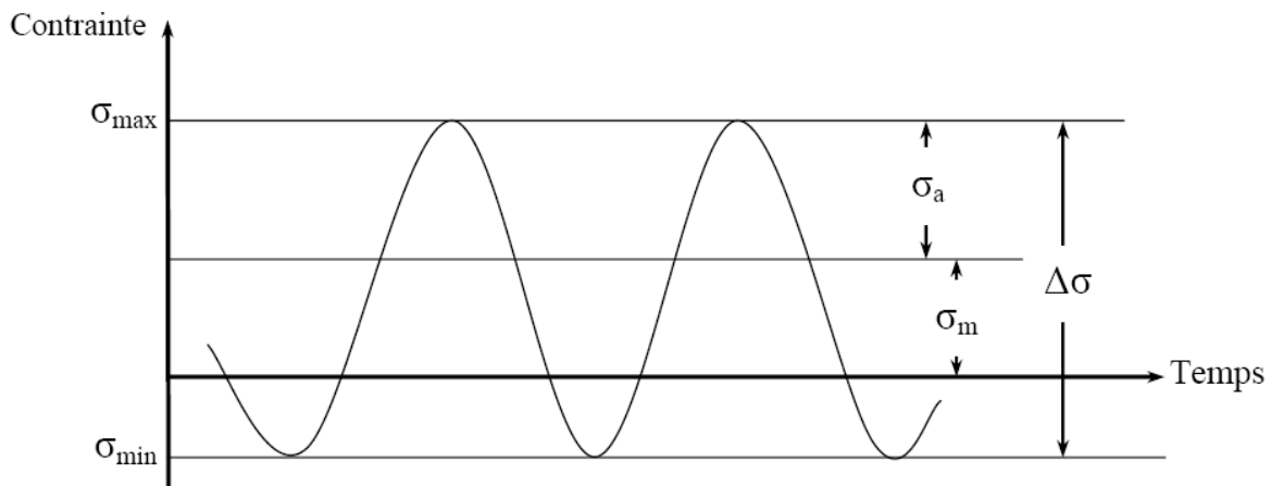
Figure I.3 : L'amplitude de contrainte.
