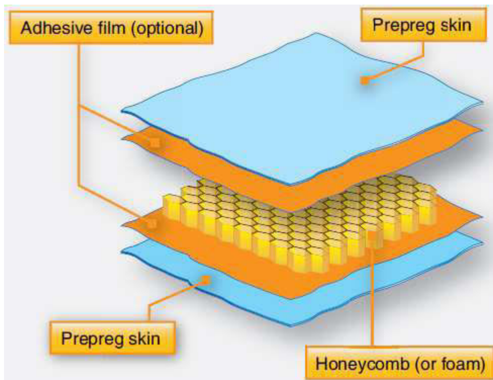
Figure II.7 : Représentation schématique des différents constituants de la structure sandwich.
