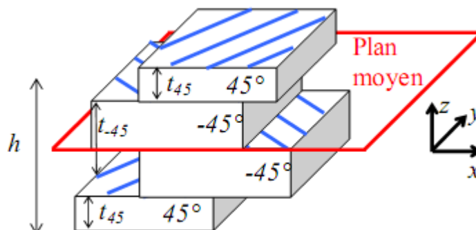
Figure II.6 : Représentation schématique d'un stratifié symétrique et équilibré
