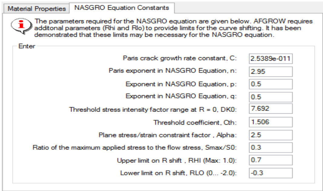
Figure III.1: Les différents paramètres de l'équation de Nasgro
