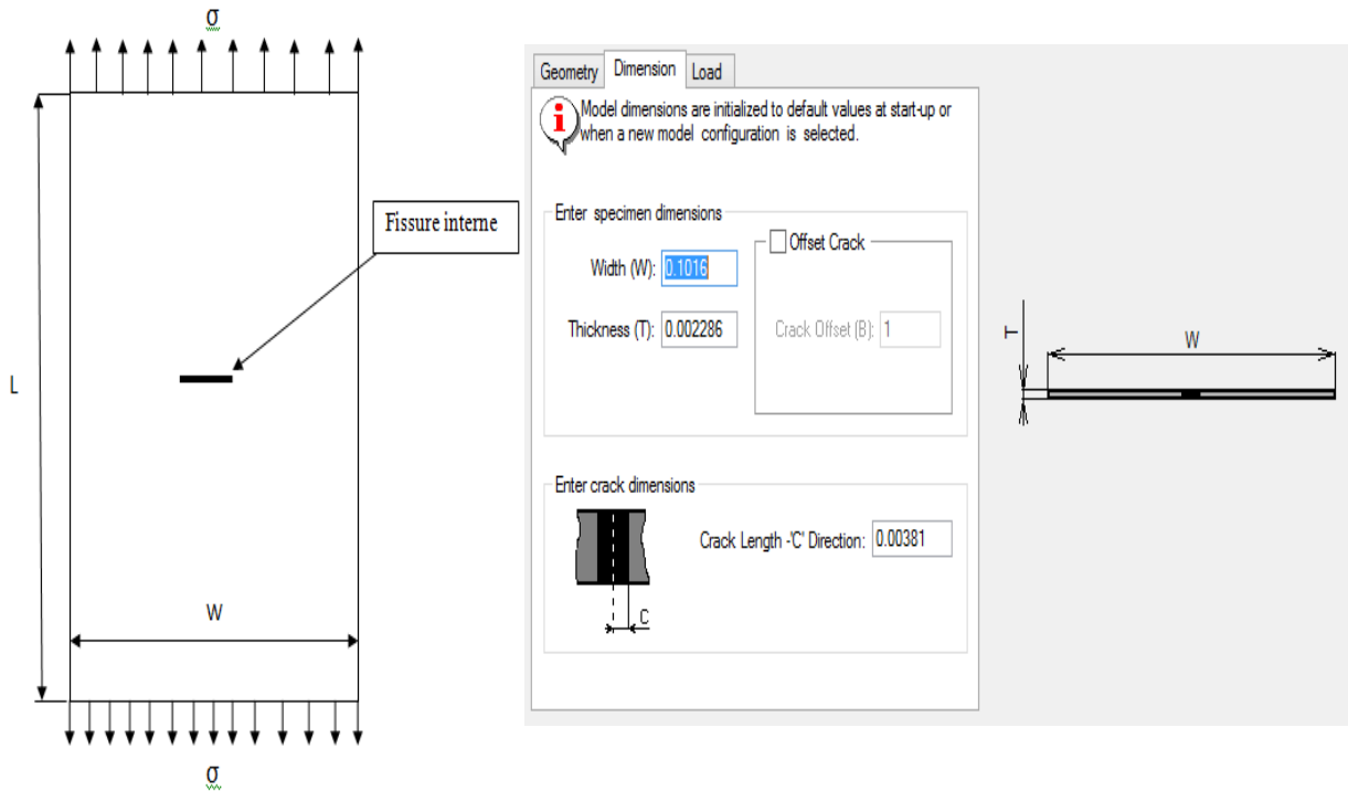
Figure III.2: Présentation du modèle.
