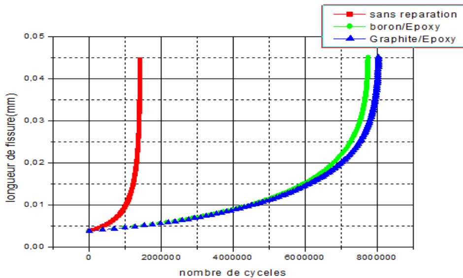
Figure III.16: Variation de la propagation de fissure en fonction du nombre de cycles de la plaque non réparée et réparée par le Bore/Epoxy et le graphite/Epoxy pour P=40 MPa.
