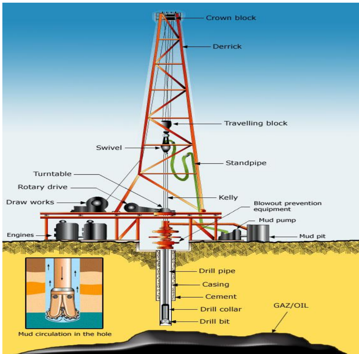
FigureI.1: Système de forage classique
