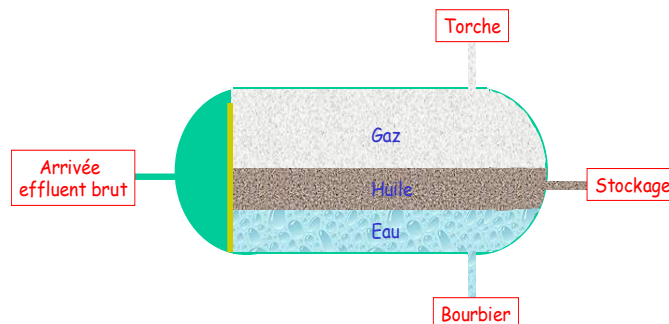
Figure I.12 : Séparateur boue-gaz
