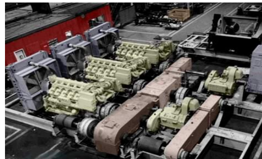
Figure I.15 : La transmission mécanique
