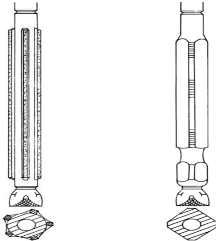
Figure I.18 : Les tiges de forage
