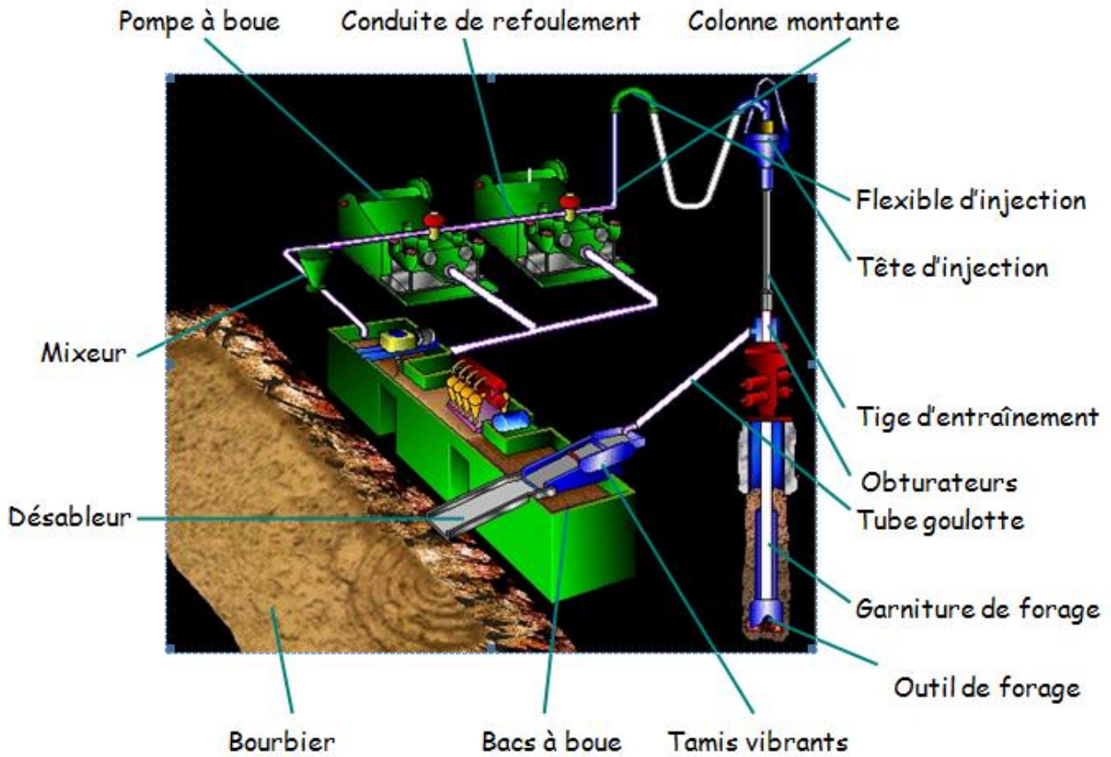
Figure I.9 :Le circuit de la boue
