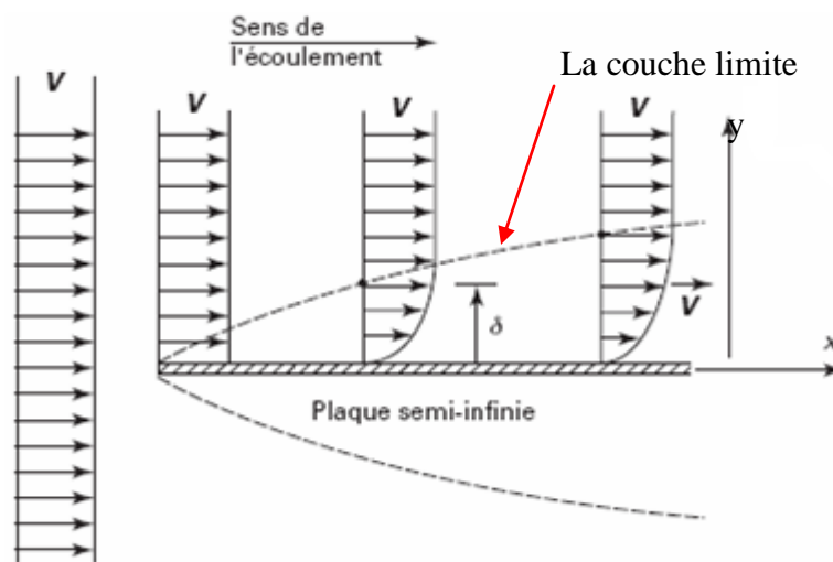
Figure III.1 : Développement d'une couche limite au voisinage d'une paroi
