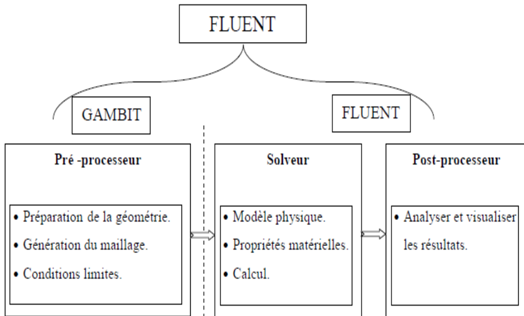
Figure III.3 : Structure de base du code "FLUENT"
