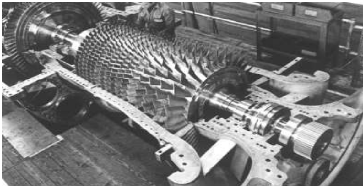
Figure 1 : Compresseur axial.
