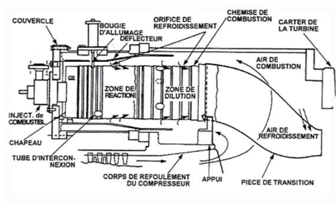
Figure 2 : Chambre de combustion.
