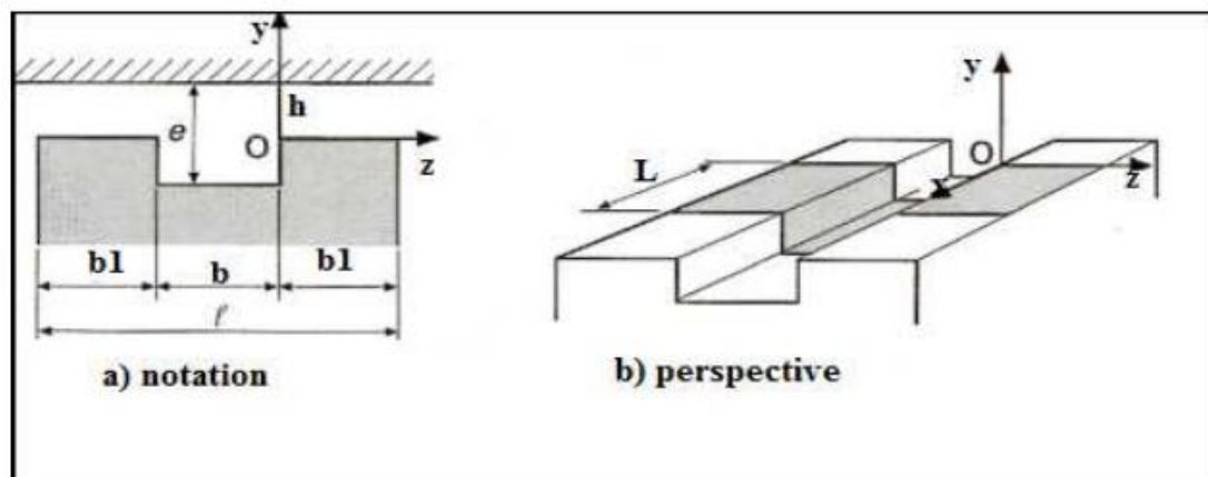
Fig. II.5 Butée hydrostatique infiniment longue n° i, a) notation, b) perspective.
