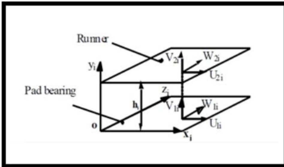
Fig. II.3 Les conditions aux limites de palier hydrostatique
