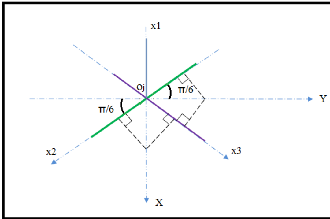
Fig. II.4 Système de coordonnées de l'arbre dans le palier
