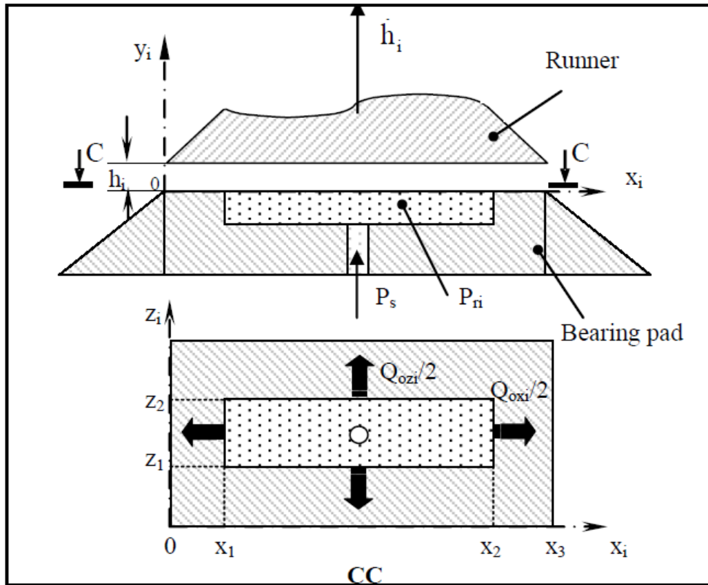
Fig. II.2 Patins de palier hydrostatique plat
