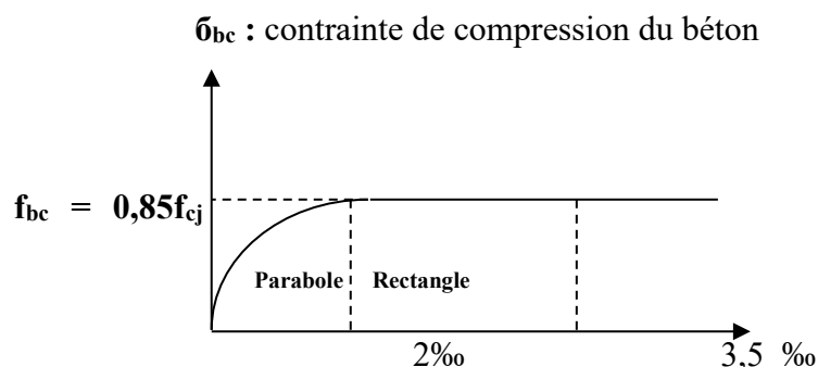
Figure I.3 : Diagramme Parabole – Rectangle.
