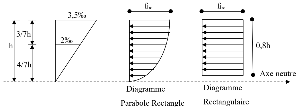
Figure I.4 : Diagramme rectangulaire.
