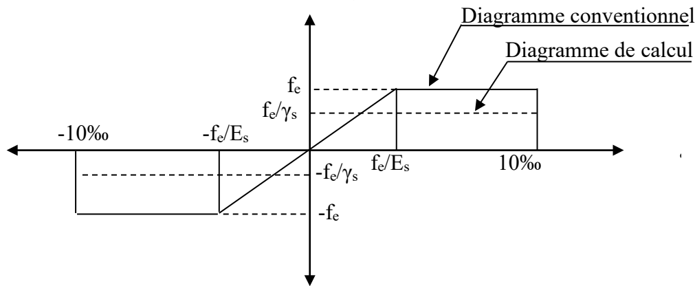
Figure I.5 : Diagramme de déformation – contraintes.
