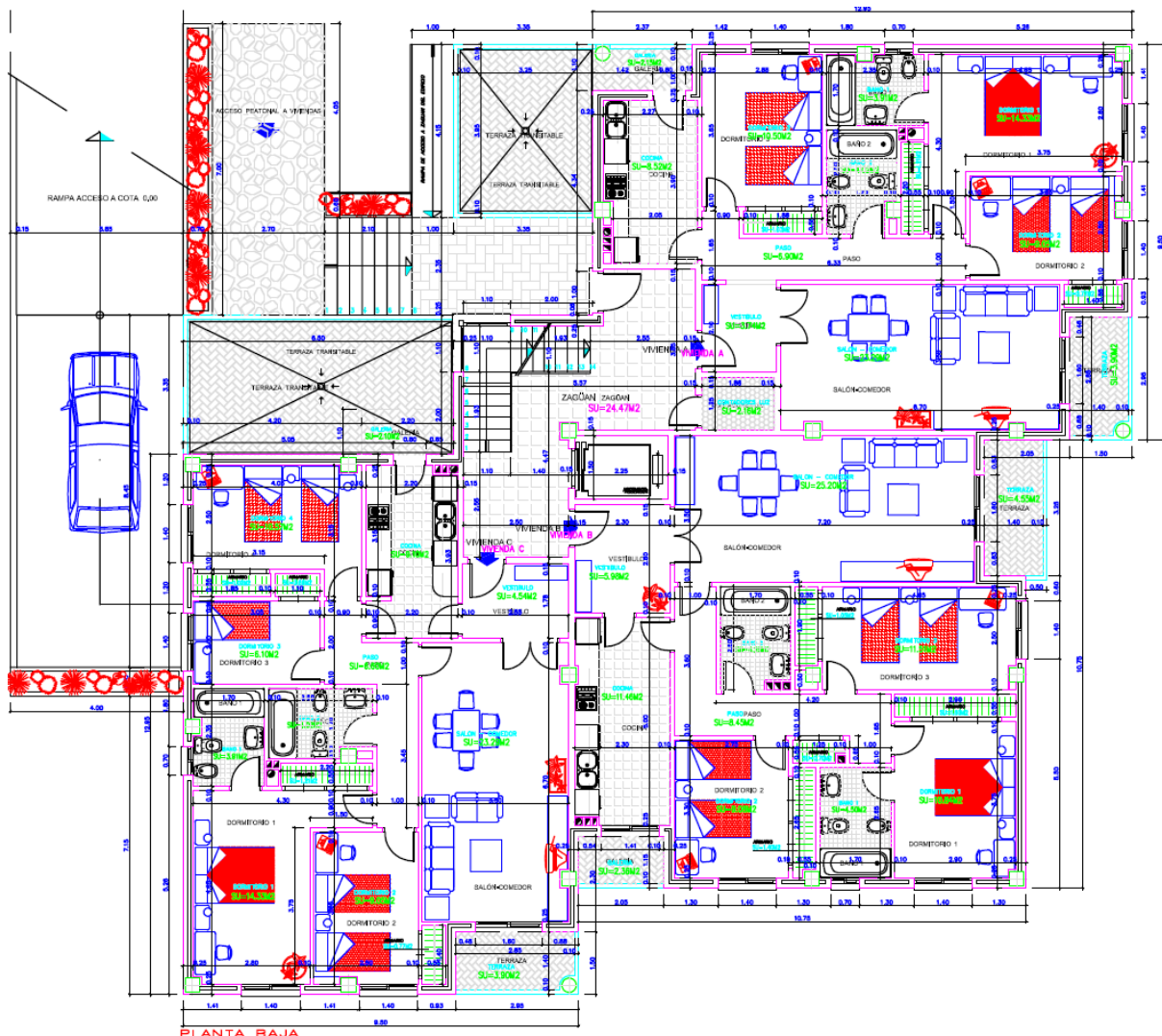
Figure I.2 : Plan étages courants
