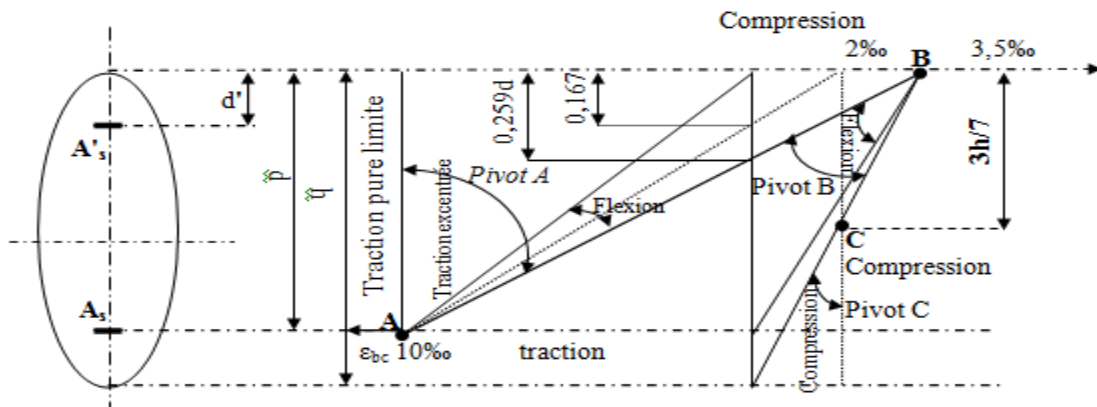
Figure I.6 : Diagramme des déformations limitées de la section.
