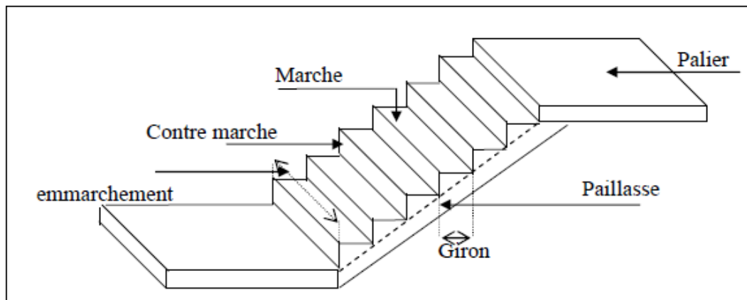
Fig. III. 12: Schéma descriptif d'un escalier.
