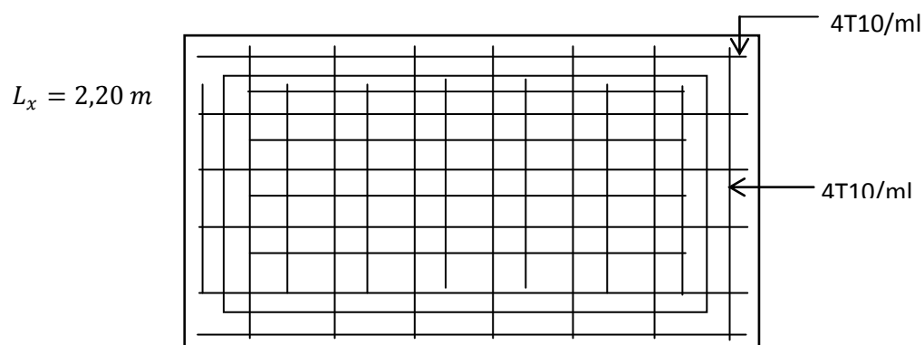
Fig. III.11 : Ferrailage inférieur de la dalle de l'ascenseur
