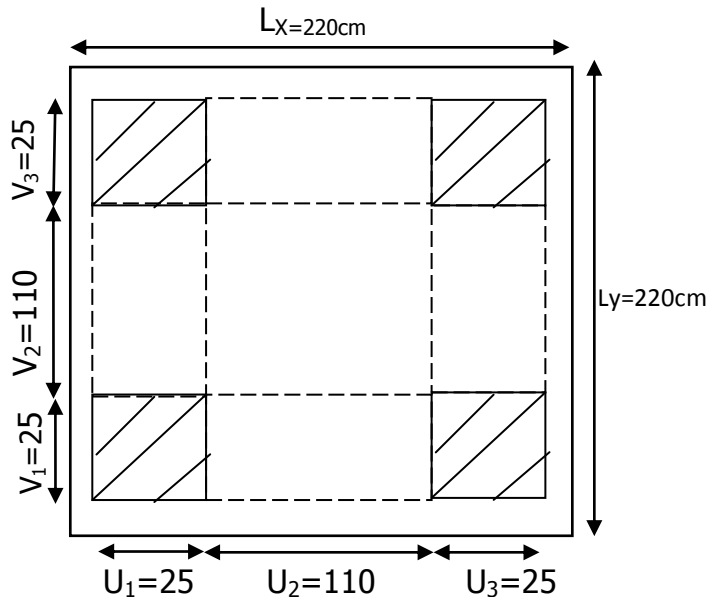
Fig. III. 8 : Dessin montrant la concentration des charges
