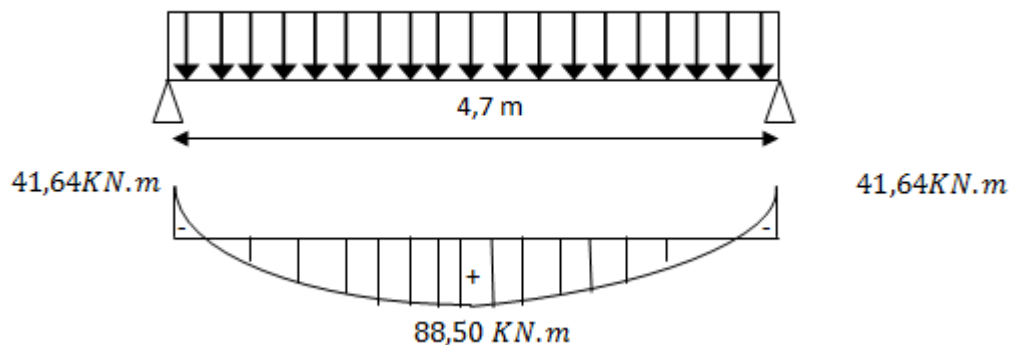
Fig. III.16 : Schéma statique de la poutre palière de l'escalier
