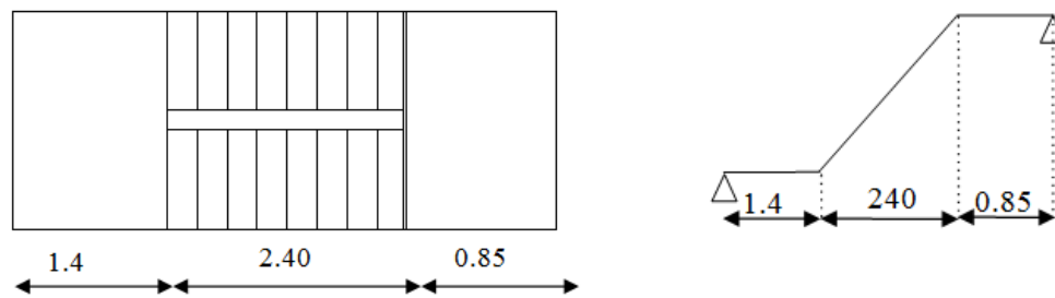
Fig. III. 13: Escalier à deux volées
