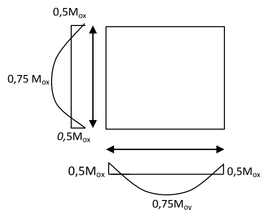
Fig. III. 9: Moments de la dalle
