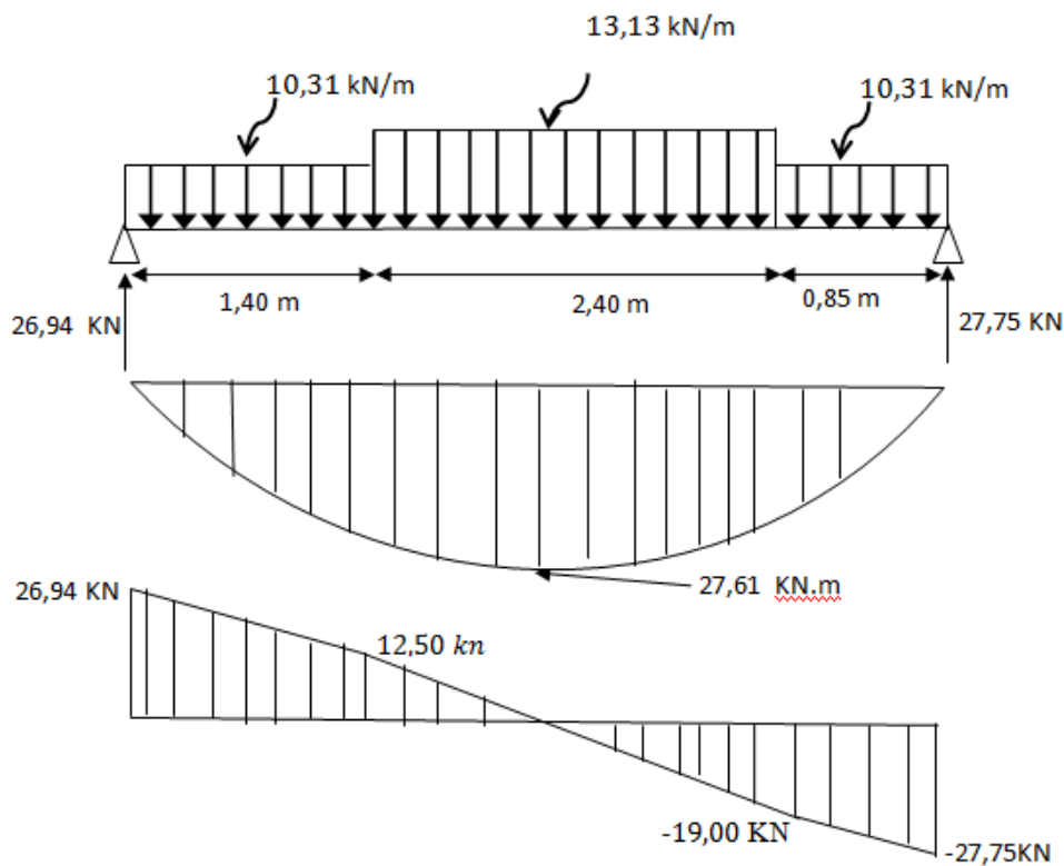
Fig. III. 15 : Diagrammes Moments et efforts tranchant (M, T) de l'escalier
