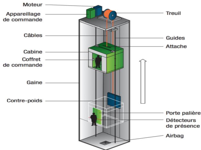
Fig. III.5: Schéma d'un ascenseur,
