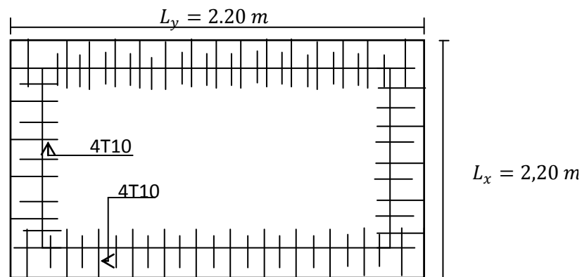
Fig. III. 10 : Ferrailage supérieur de la dalle de l'ascenseur,
