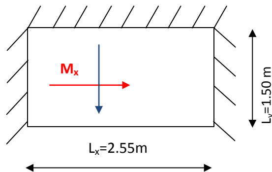
Fig. III. 1 : Schéma de type du balcon
