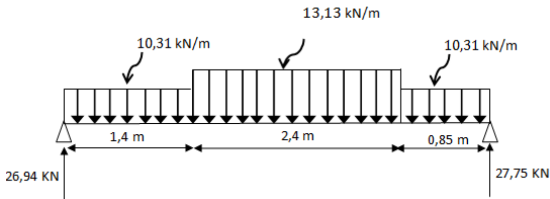
Fig. III. 14: Schéma statique de l'escalier
