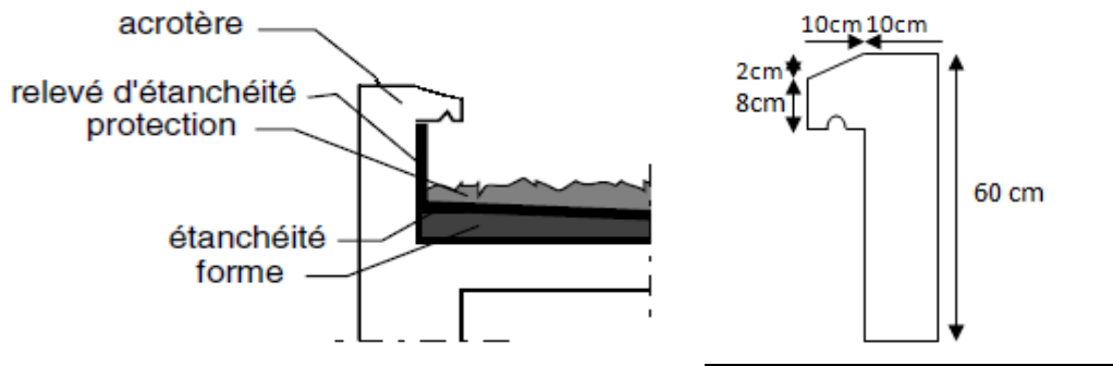
Figure. III.3 : Acrotère en béton armé.
