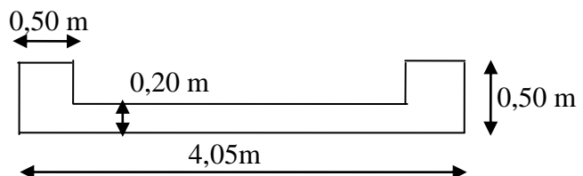
Figure-VIII -1: Schéma de voile
