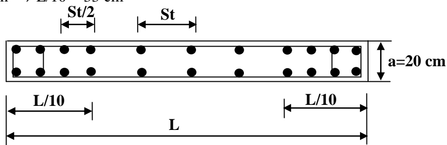
Figure -VIII-2:Disposition des armatures verticales dans les voiles
