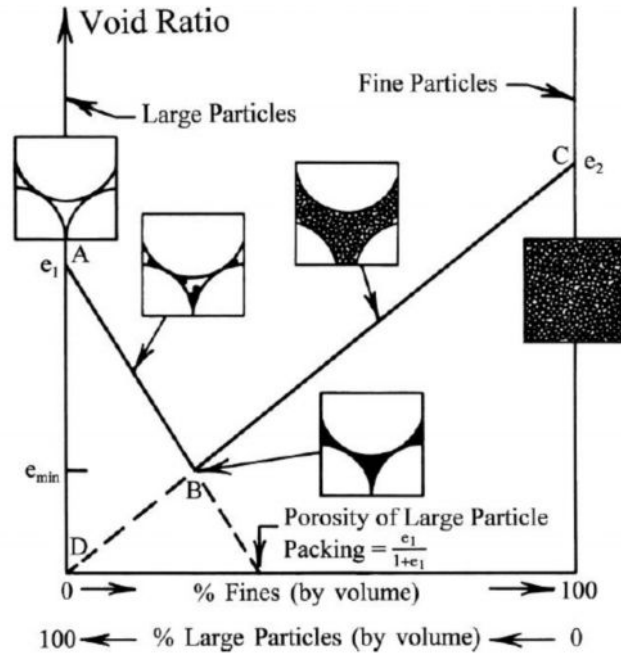
Figure II.1: Diagramme schématisant des valeurs limites de la teneur en fines (Lade, 2012)
