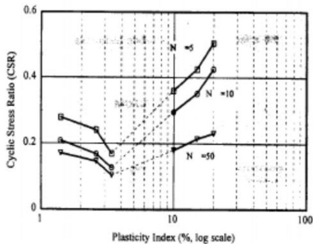
Figure II.14: Variation de la résistance à la liquéfaction en fonction de l'indice de plasticité (Tianqiang et Prakash, 1999).
