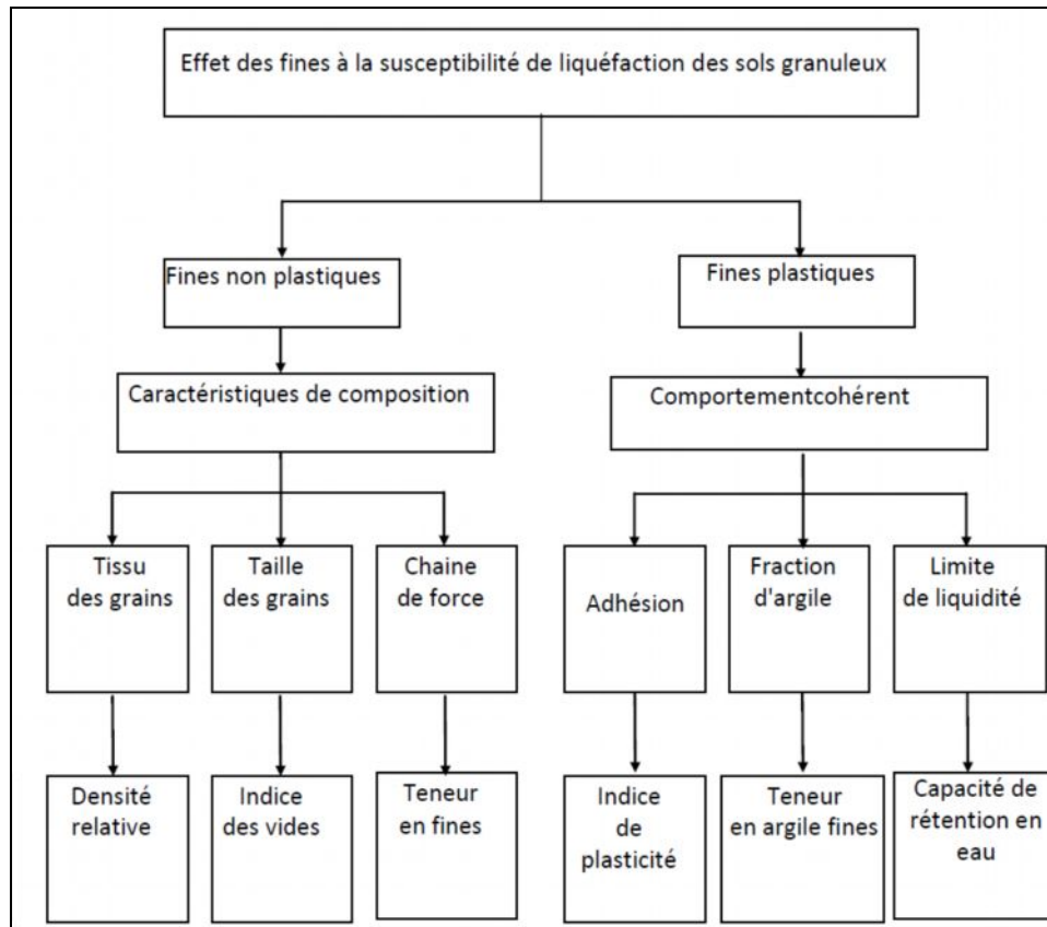
Figure II.3: Vue d'ensemble du rôle des fines à la susceptibilité de liquéfaction des sols
