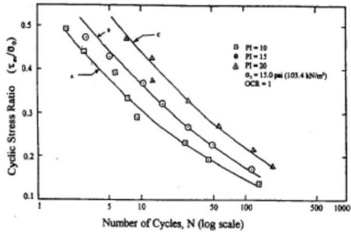
Figure II.13: Influence de l'indice de plasticité sur la résistance à la liquéfaction (Puri 1984).
