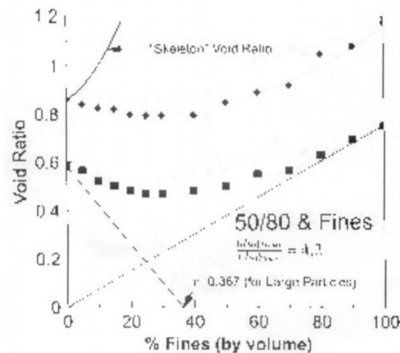
Figure II.7: Variation de l'indice des vides en fonction de la teneur en fines (Lade et Yamamuro, 1998).
