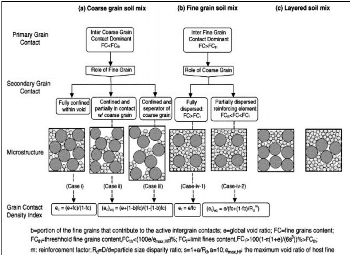
Figure II.4: Classification de tissu de grain dans les sols de la matrice de sable (Thevanayagam et Martin, 2002)
