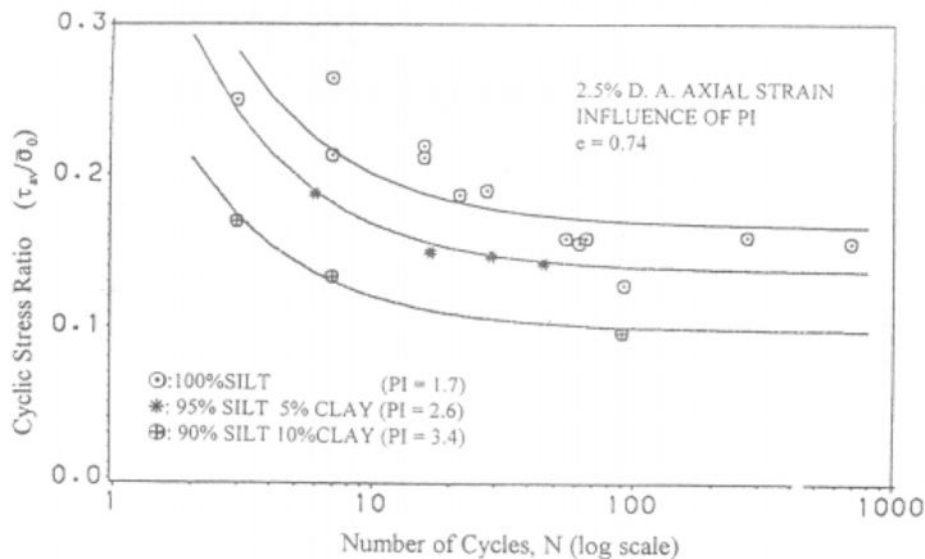
Figure II.12: Influence de l'indice de plasticité sur la résistance à la liquéfaction (Sandoval 1989; Prakash et Snadoval, 1992).
