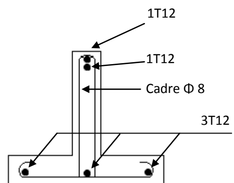
Appui intermédiaire
