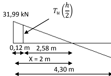
Figure .IV.1: Effort tranchant par la méthode des triangles semblables.
