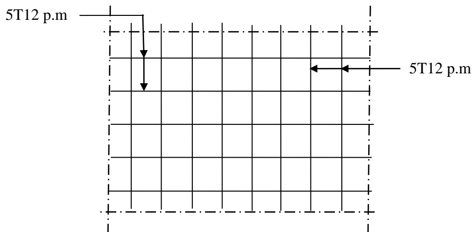
Figure.8.2- Disposition du ferrailage du voile.
