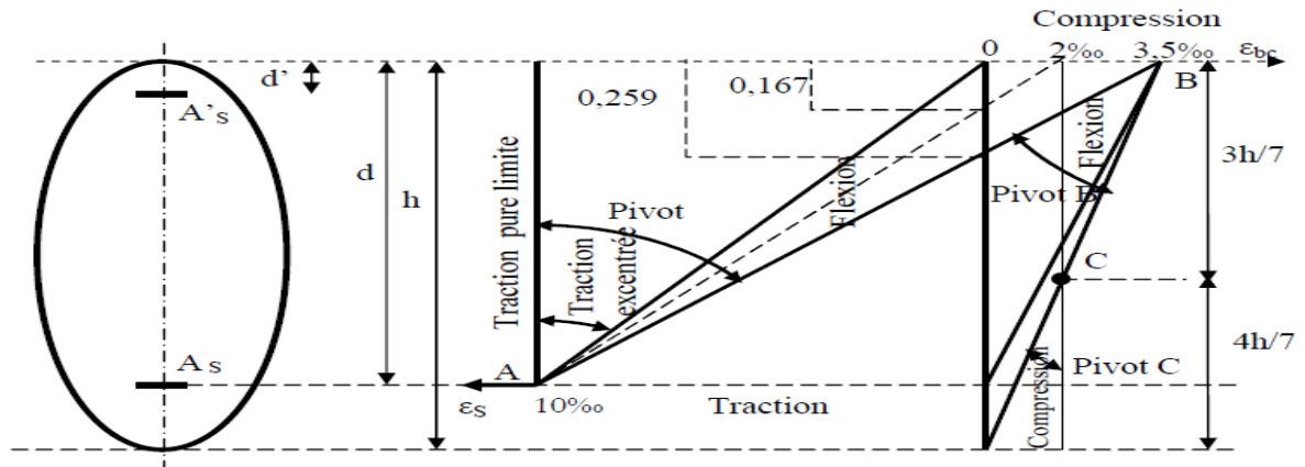
Figure I.4 : Diagramme des déformations limitées de la section.
