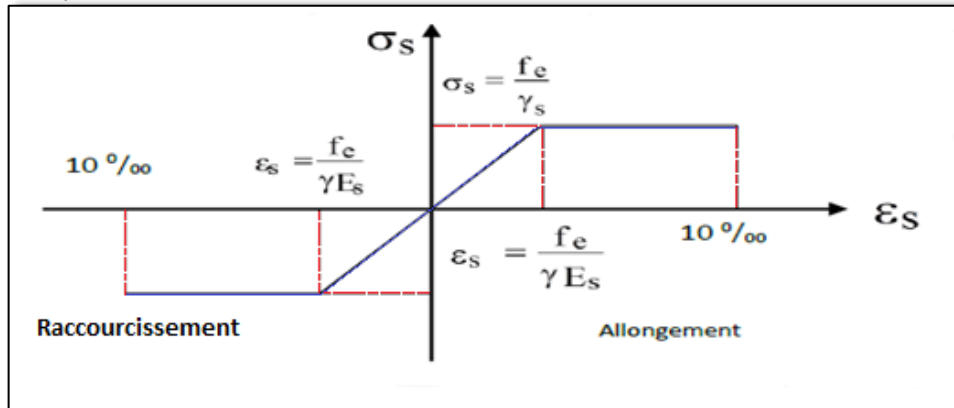
Figure I.3 : Diagramme de déformation – contraintes.
