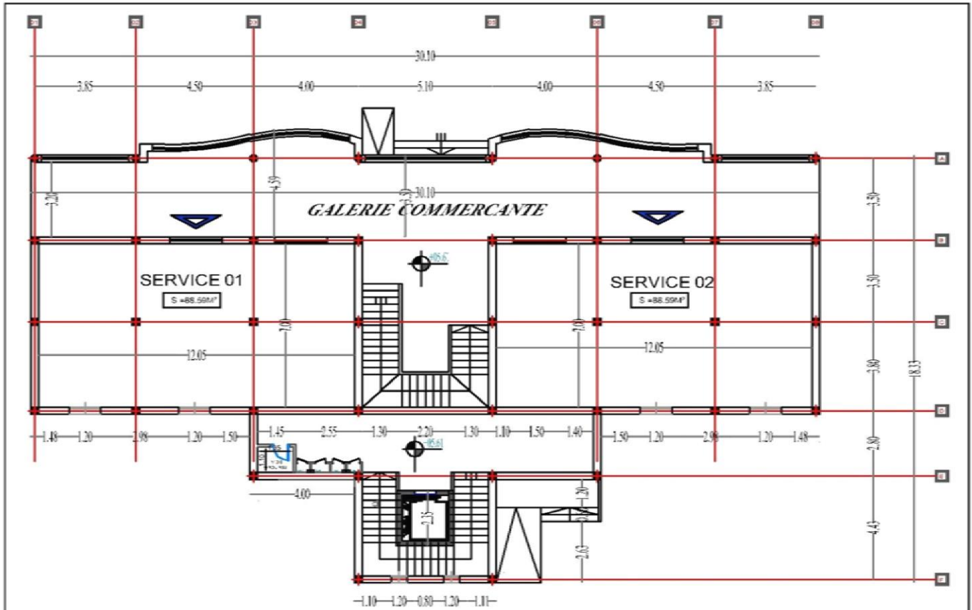
VUE EN PLAN DU 1er ETAGE
