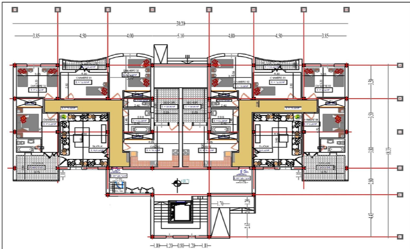
VUE EN PLAN DU 2 eme ETAGE
