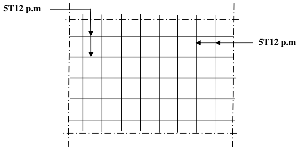
Figure VII-2- disposition du ferrailage du voile
