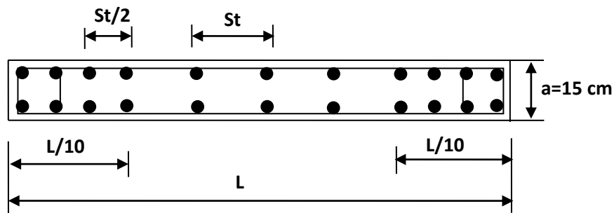
Fig.VII.1.Disposition des armatures verticales dans les voiles
