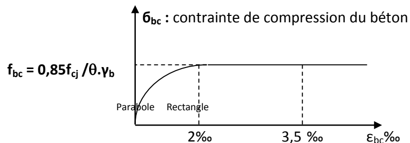
Figure I.1- Diagramme de déformations – contraintes
