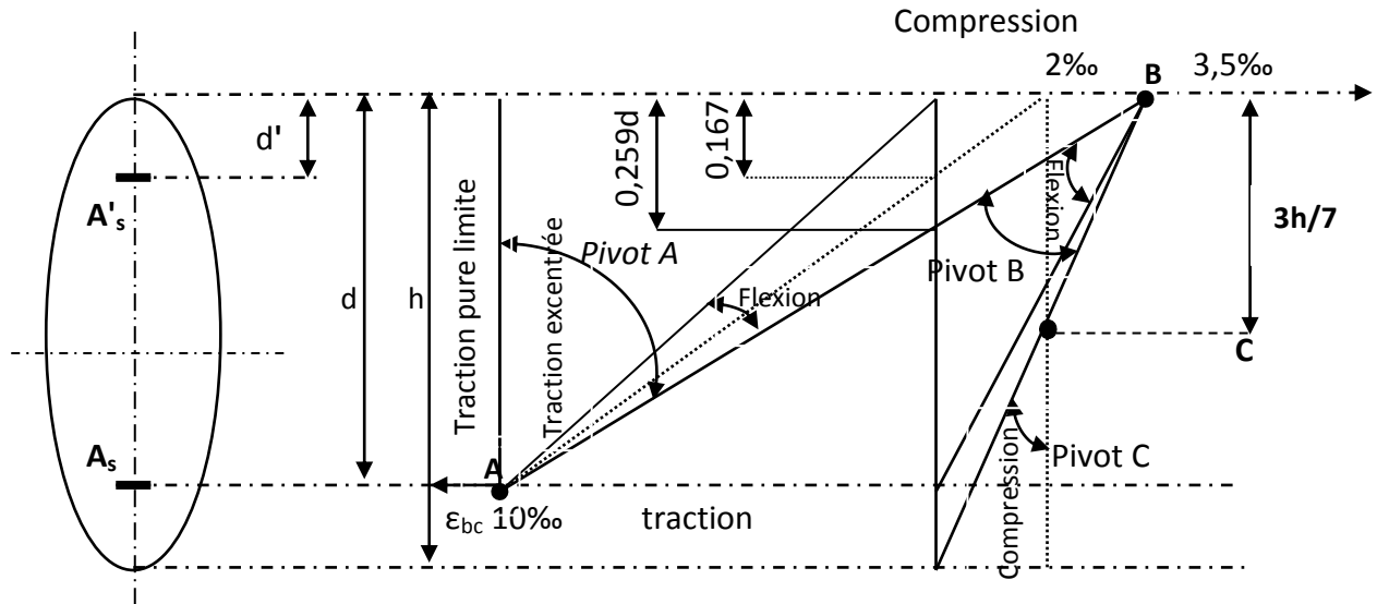
Figure I.4- Diagramme des déformations limitées de la section
