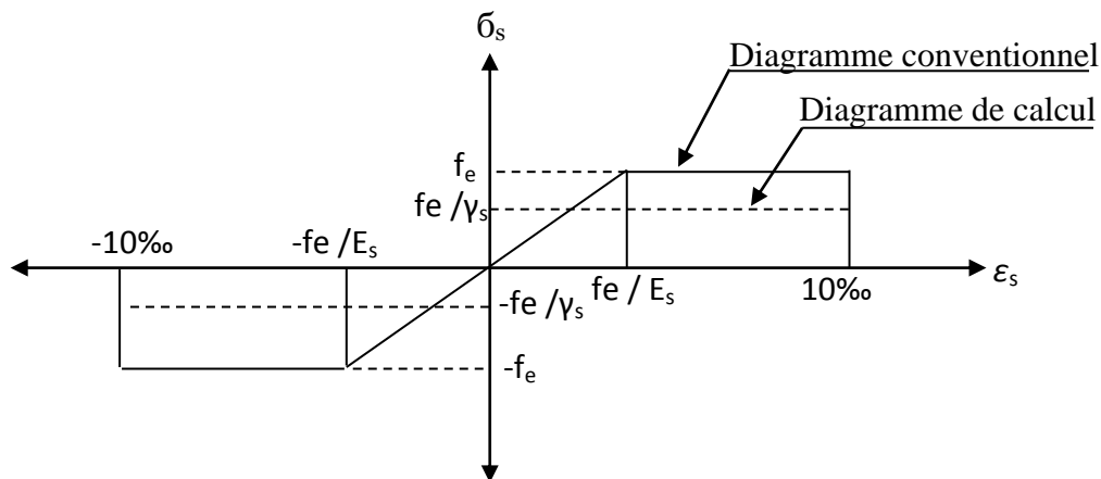
Figure I.3- Diagramme de déformations – contraintes.
