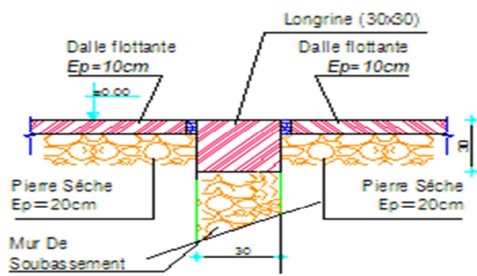
Coupe B- B
