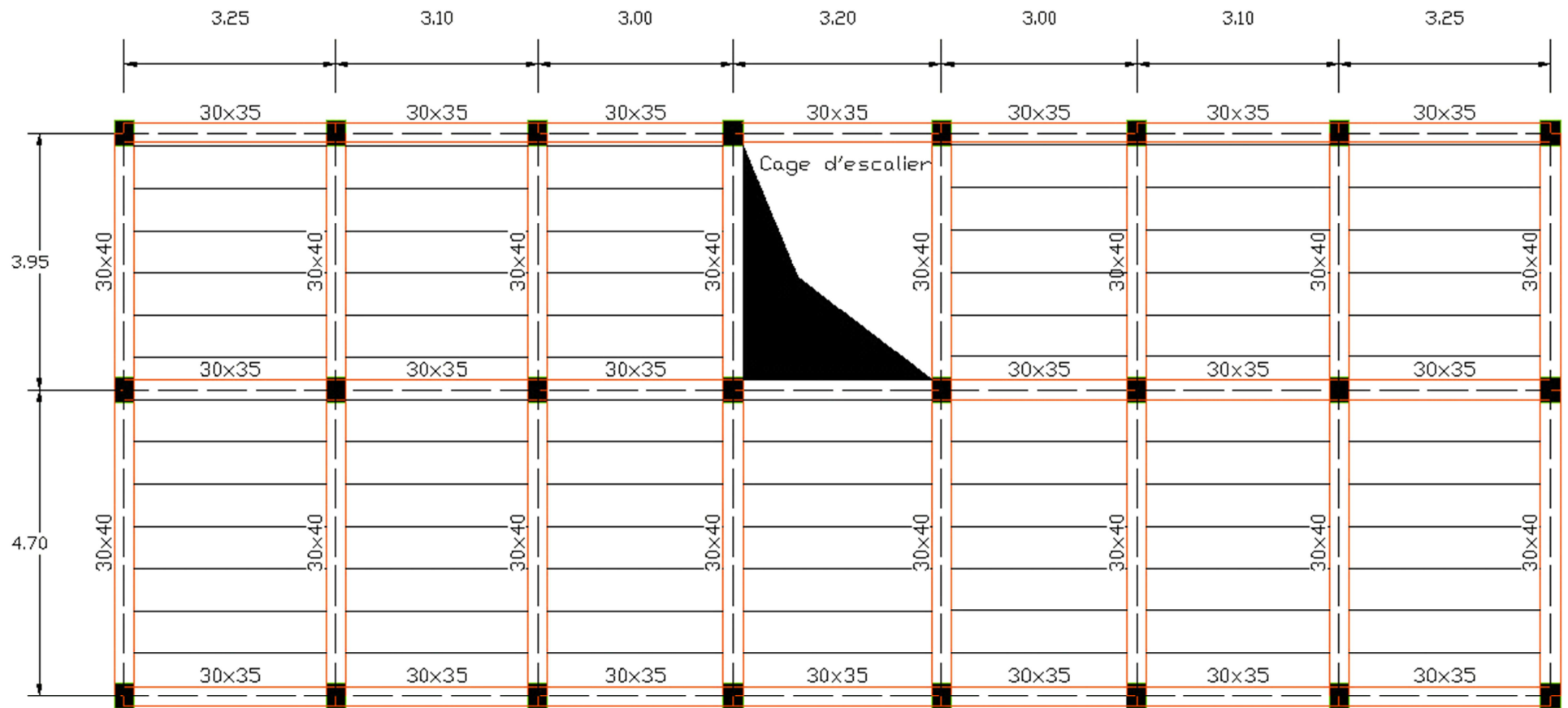
Plan De Coffrage Planche Etage Courante
