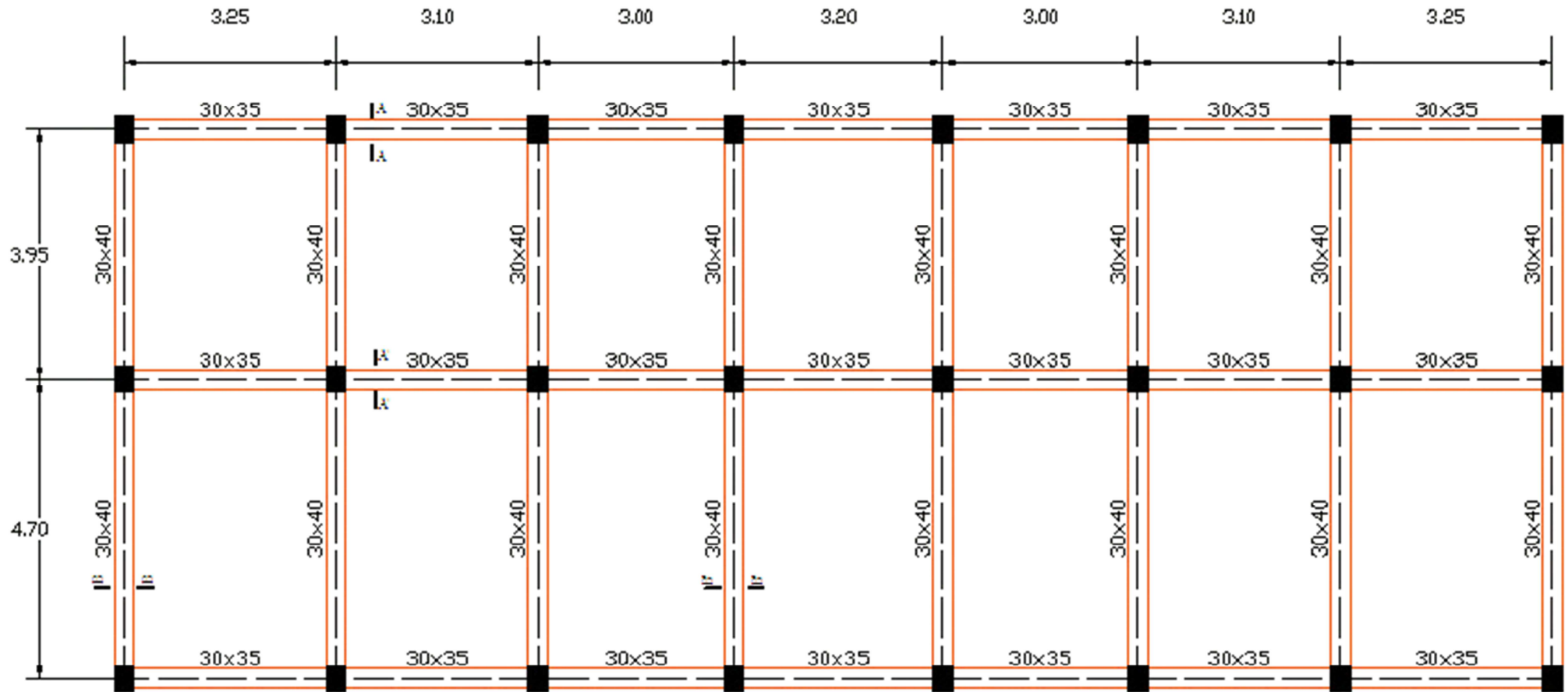
Plan De Coffrage Plancher Terrasse
