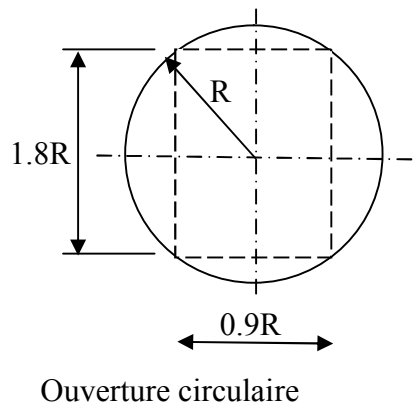
Fig.1.5: configuration de la poutre avec l'ouverture
