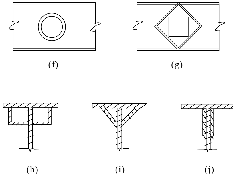
Fig.1.7 : renforcement de l'ouverture
