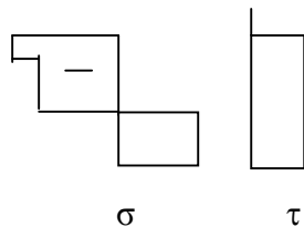
Fig.1.6: distribution des contraintes plastiques.
