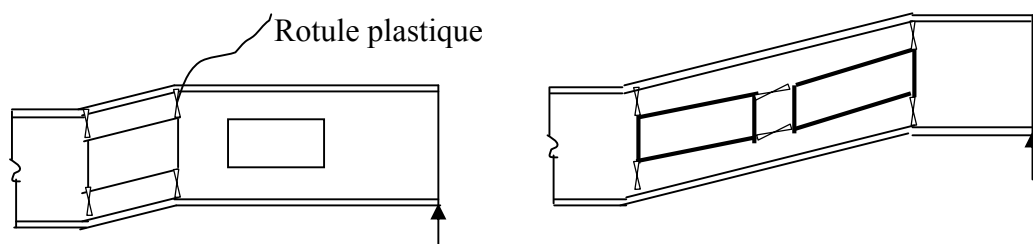
(a) une seule ouverture et modes interactifs de ruine.
