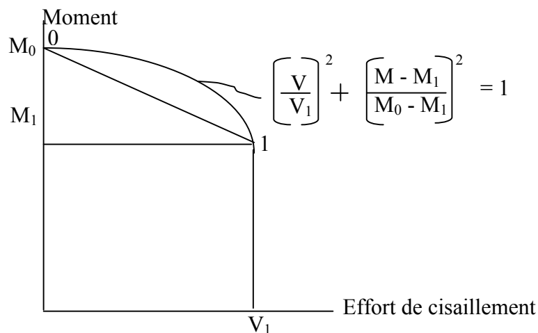
Fig. 1.4: Diagramme d'interaction de la résistance.
