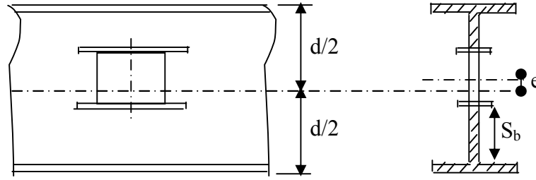
Fig.1.8 : ouverture d'une poutre métallique.
