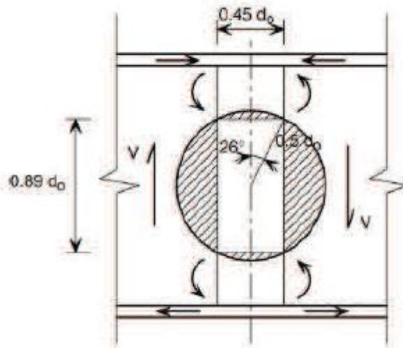
Figure 1.14 : Ouverture rectangulaire équivalente [R2]
