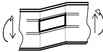
Fig.1.3: mode de ruine d'une poutre à une seule ouverture.
