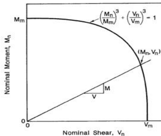
Figure 1.10 : Diagramme cubique d'interaction Moment-Effort tranchant [D2]
