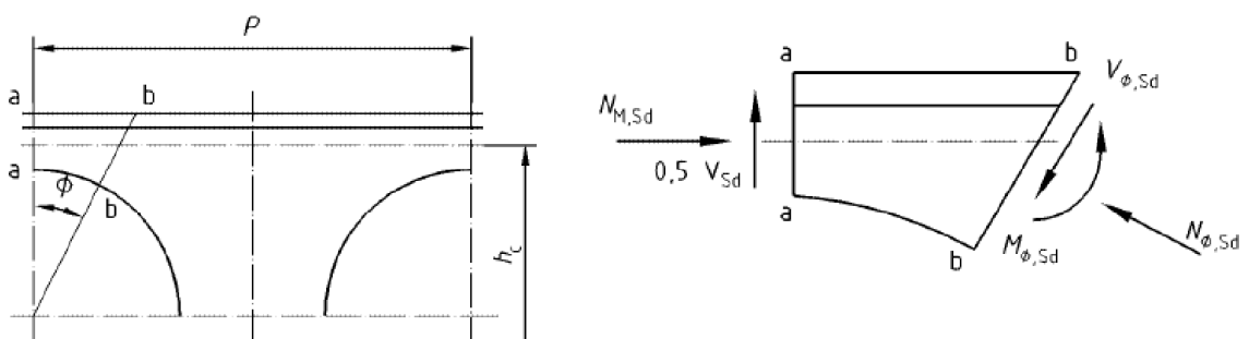
Figure 1.13 : Sollicitations sur une section plane inclinée d'un angle \phi [E2]
