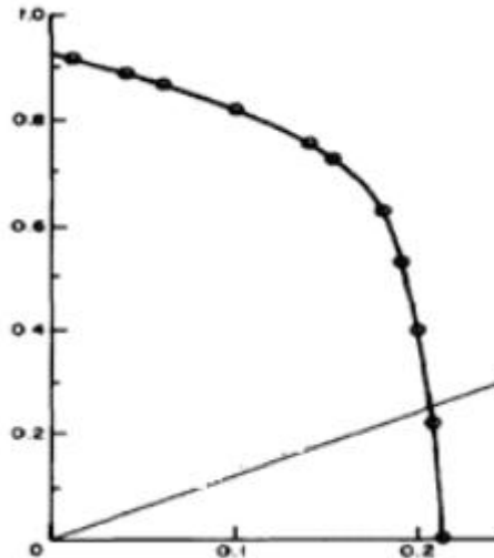
Figure 1.9 : Diagramme d'interaction construit à partir de plusieurs points
