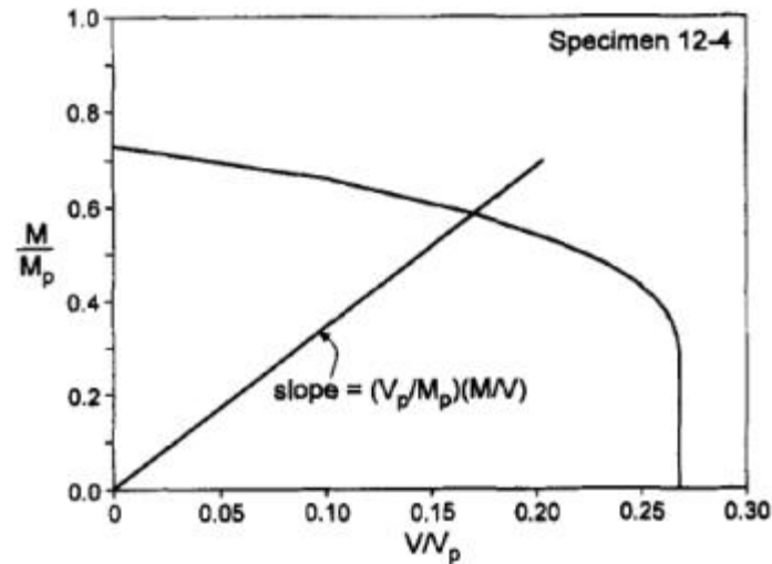
Figure 1.11 : Courbe d'interaction Moment-Effort tranchant [R4]
