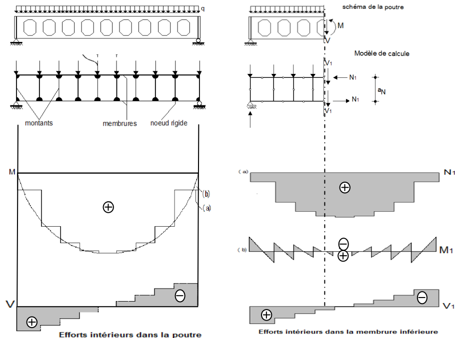
Fig. II.1 – Poutre ajourée : modèle de calcul.
